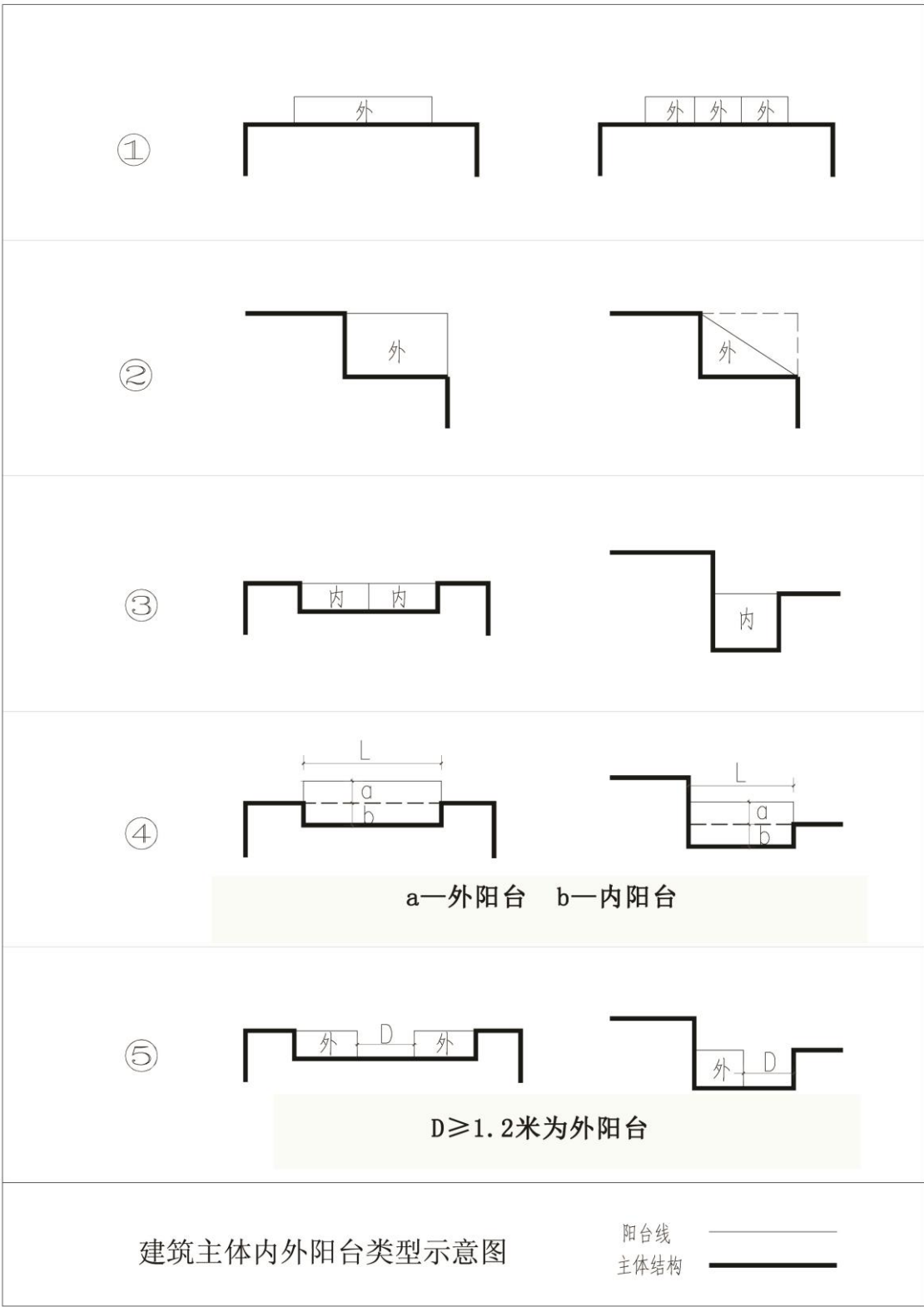
附图 1 建筑主体内外阳台类型示意图
