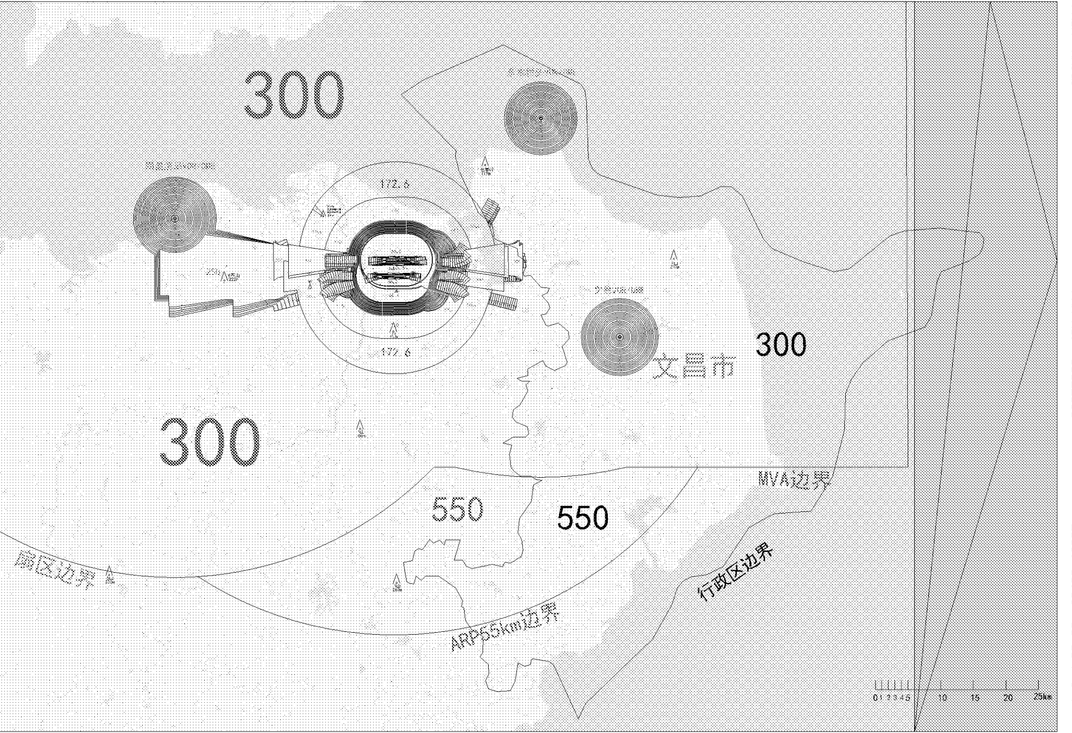
附图五：海口美兰机场飞行服务程序净空保护区一体化图（文昌市分图）
