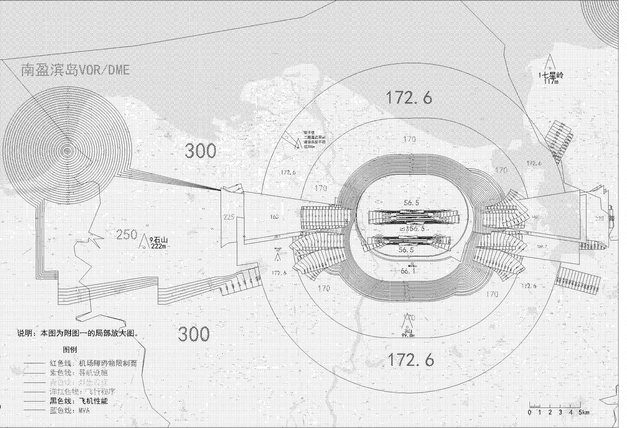
附图二：海口美兰机场航行服务程序净空保护区域一体化图（局部放大图）
