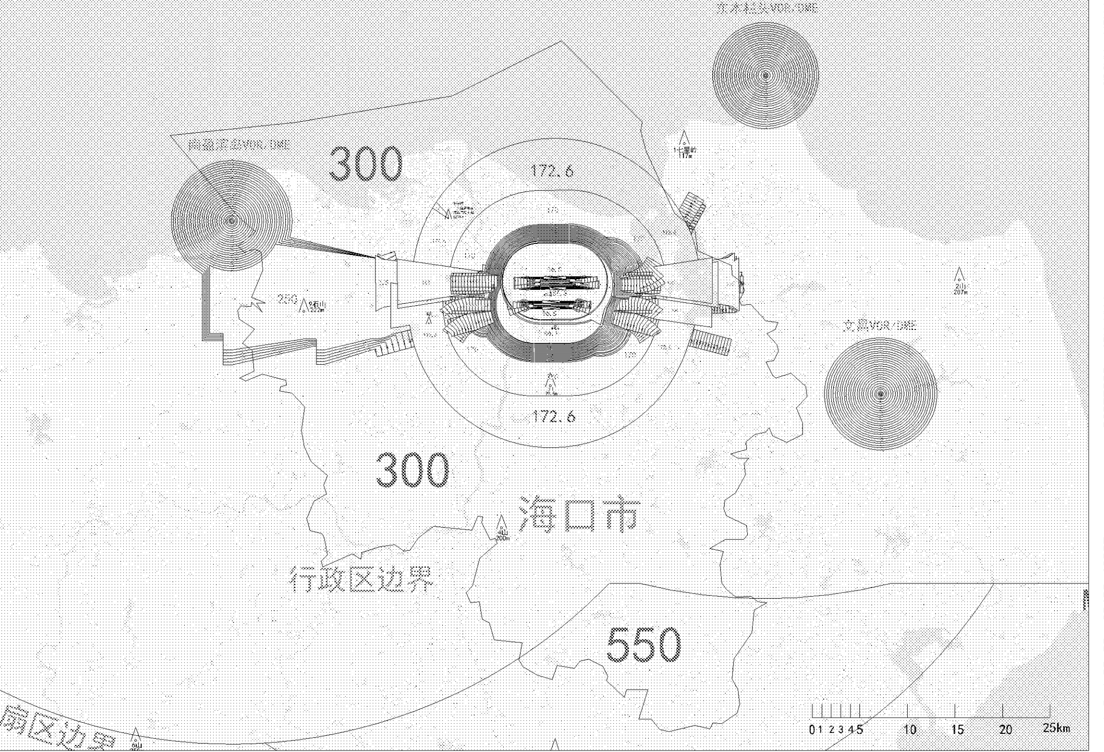
附图六：海口美兰机场飞行服务程序净空保护区域一体化图（海口市分图）
