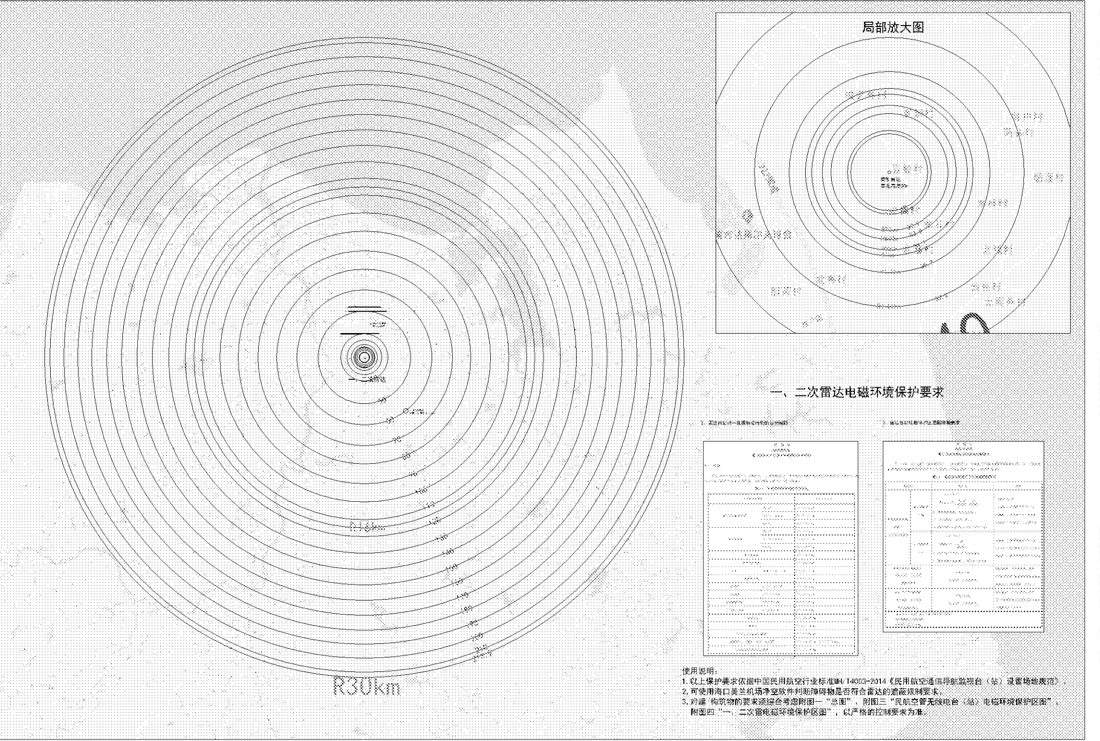
附图四：海口美兰机场一、二次雷达电磁环境保护区图
