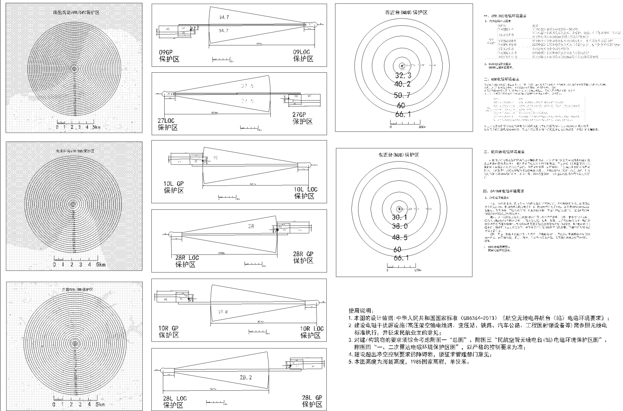
附图三：海口美兰机场民航航空管无线电台(站)电磁环境保护区图
