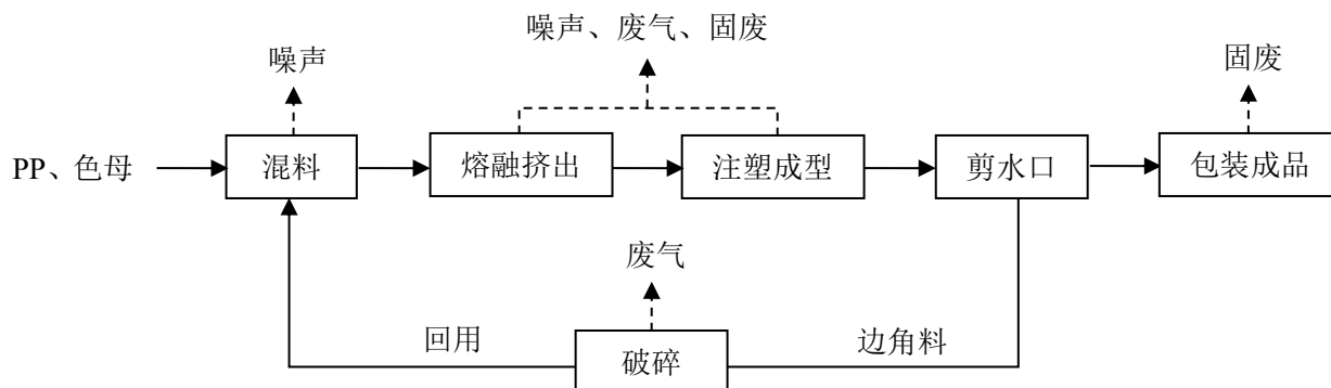
图 1 项目生产工艺流程及产污图
