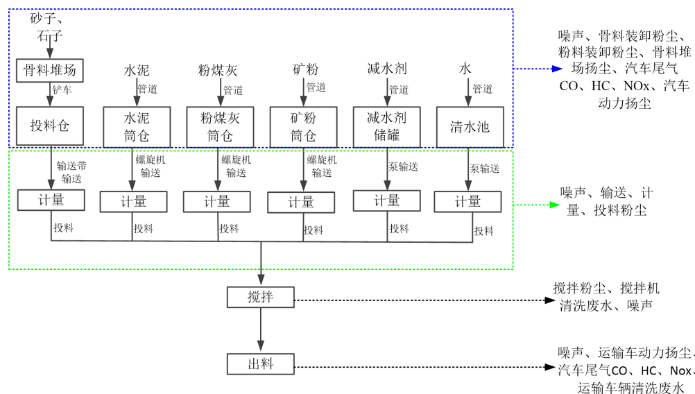
图 2-2 项目商品混凝土生产工艺流程图
