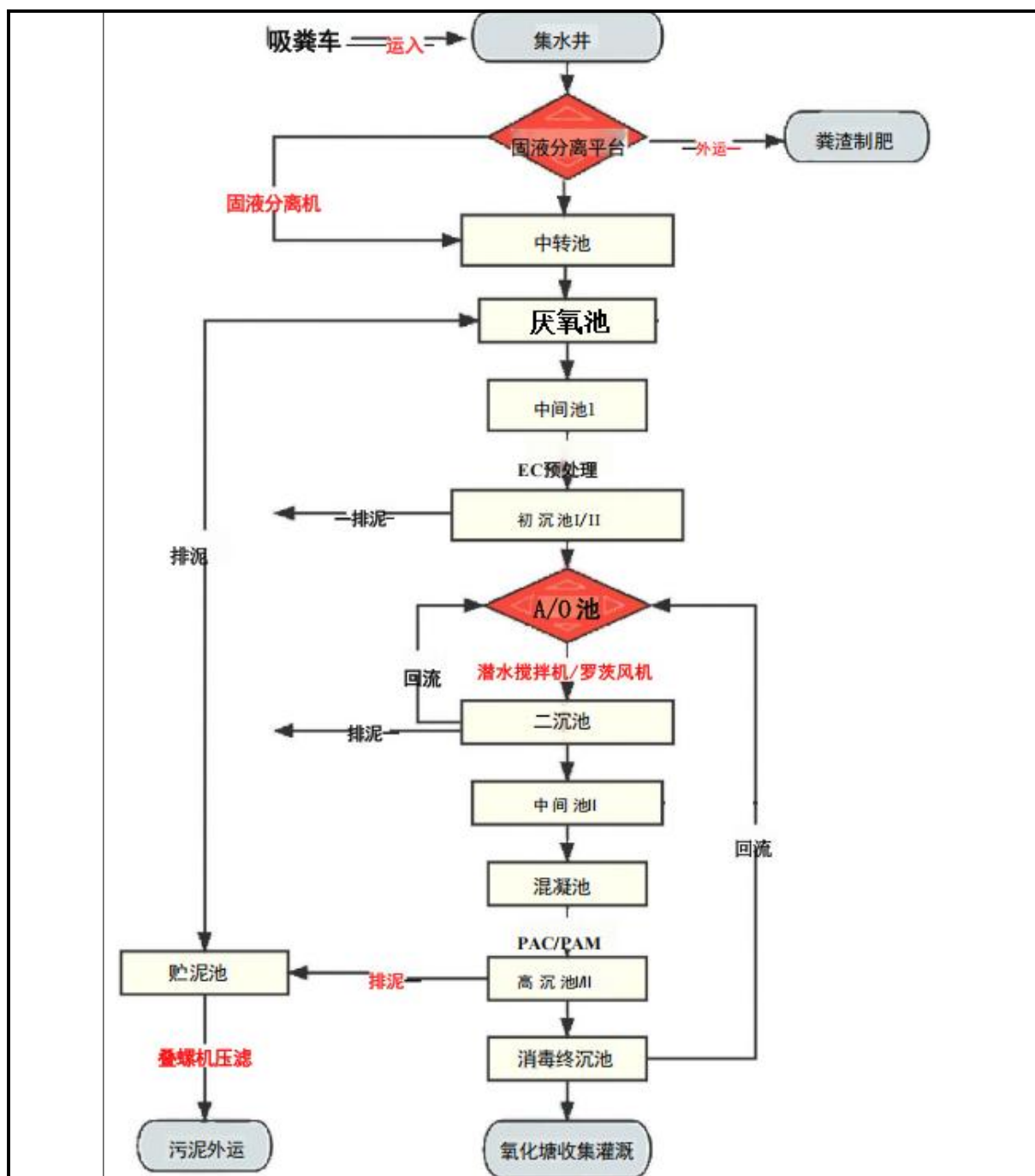
图 2-2 项目生产工艺流程及产污环节示意图
