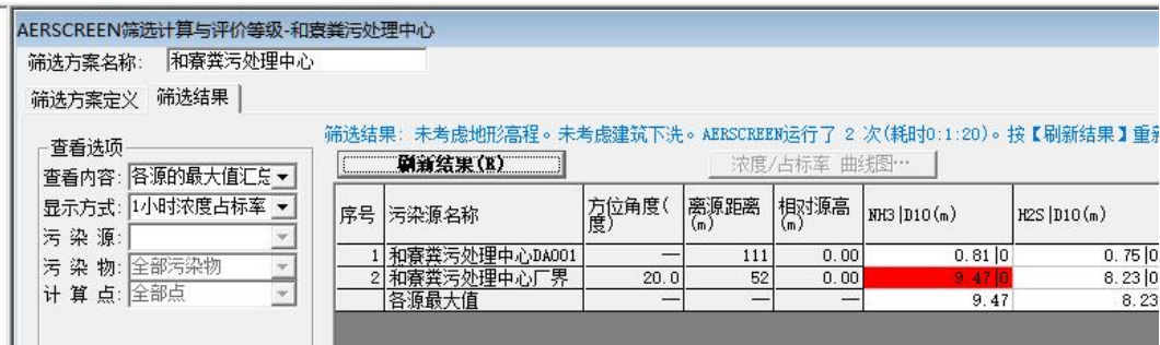
图 4-1 大气预测结果
