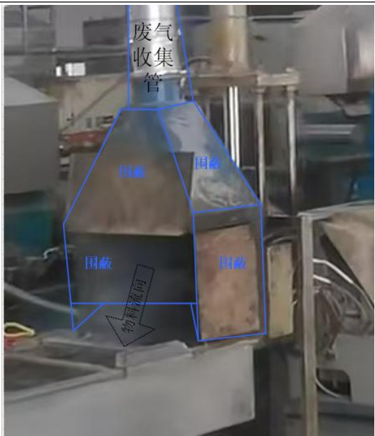
团料机集气罩示意图(非实物图，仅供参考)
