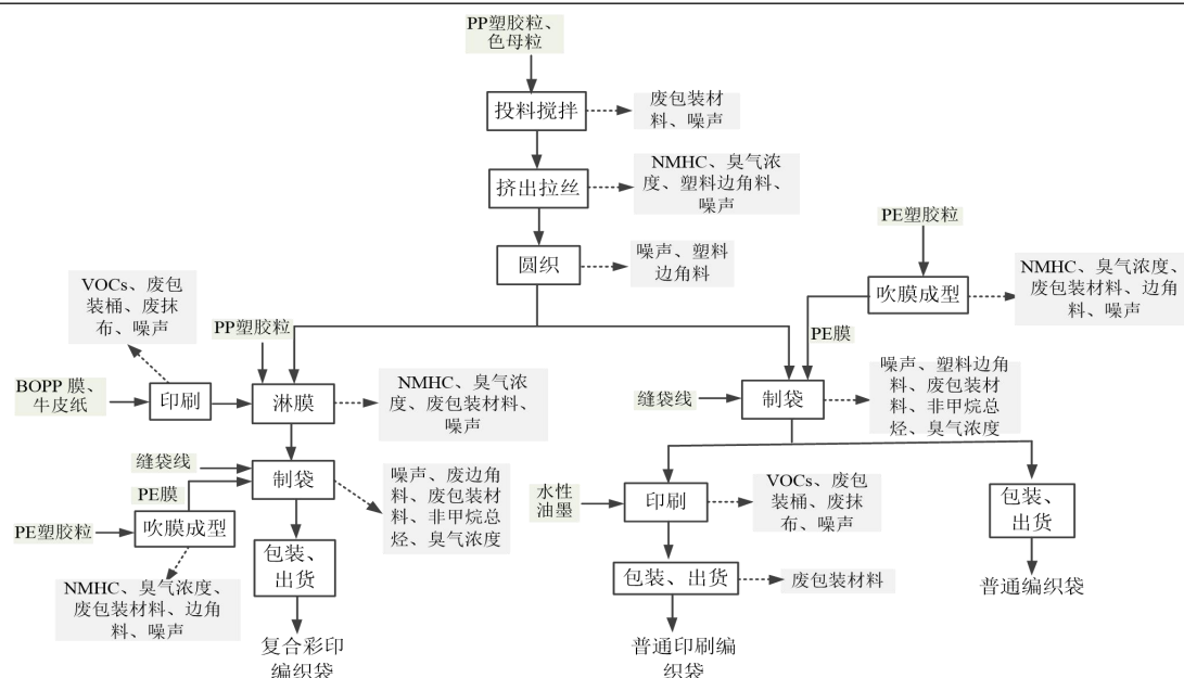
图 2-3 项目编织袋生产工艺流程图
