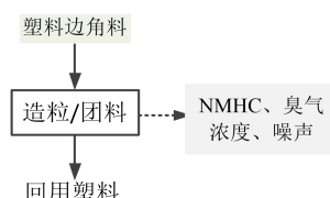
图 2-4 塑料边角料回用工艺流程图
