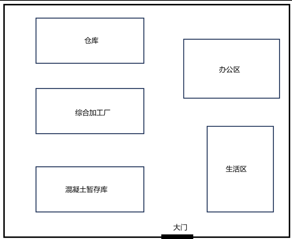
图 2-4 施工生产生活区布置示意图
