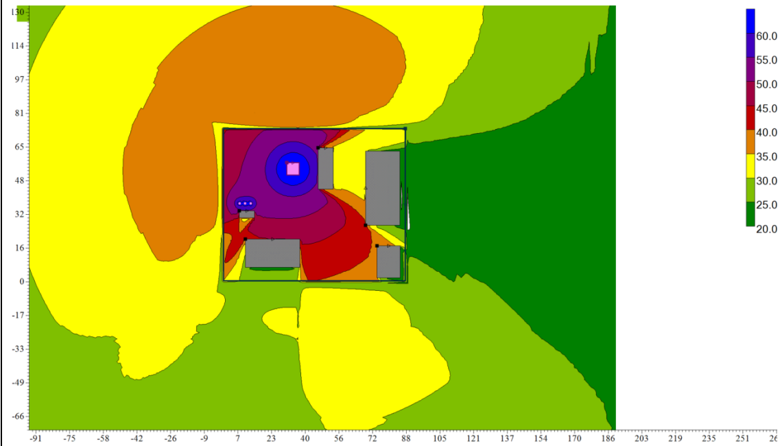
图4-7 噪声预测等值线图
