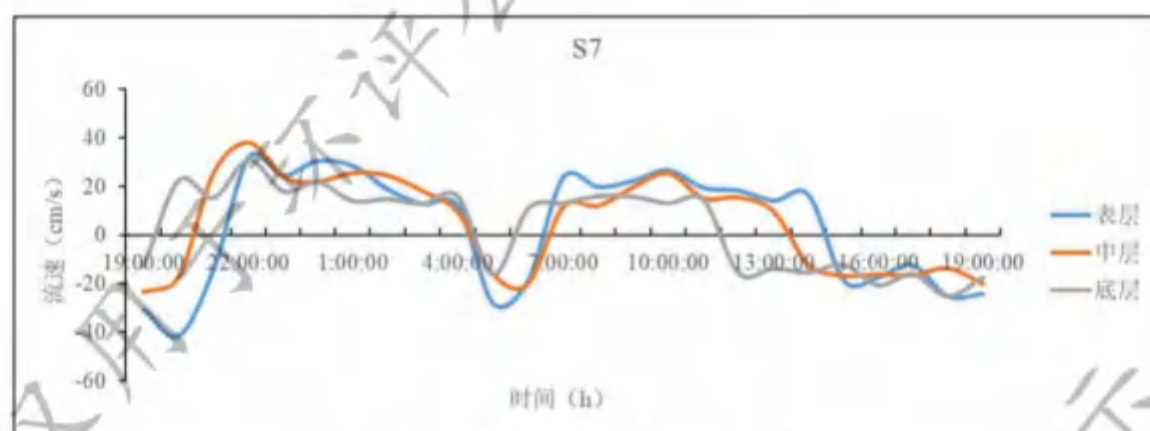
图 3-8 S7 测站实测海流流速过程图
