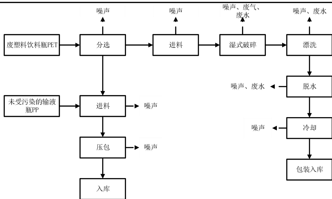
图 2-3 运营期工艺流程图
