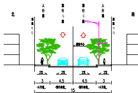
标准横断面图
