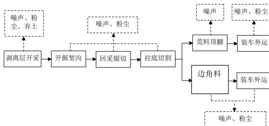
图 2-2 项目运营期工艺流程图
