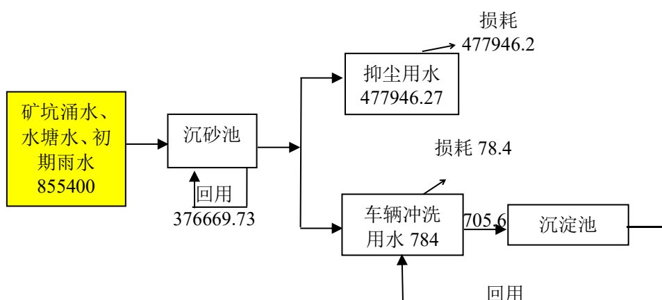
图 2-1 水平衡图 (单位: m 3 /a)
