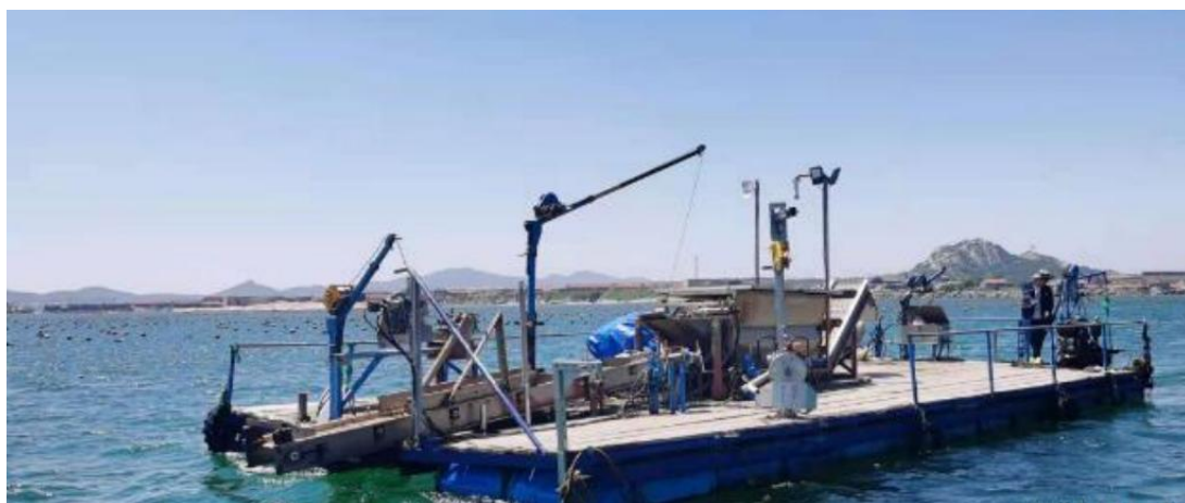
图 3.4-5 牡蛎筏式养殖的机械化采收
