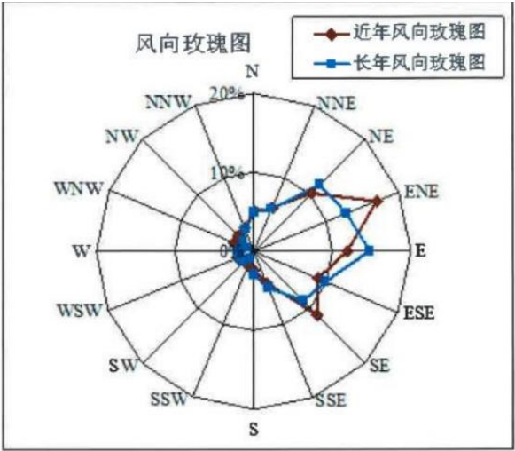
图 5.1.1-1 徐闻气象站长年及近年风向玫瑰图
