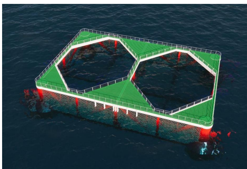
图 3.2.3-4 简易钢制网箱示意图
