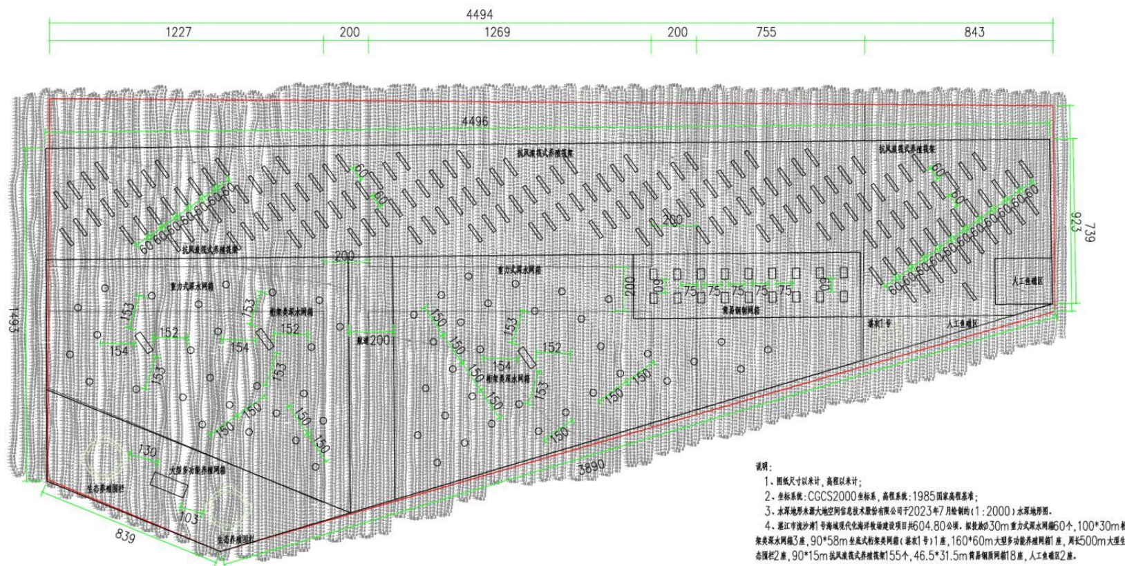
湛江市流沙湾1号海域现代化海洋牧场建设项目平面布置图 1:10000
