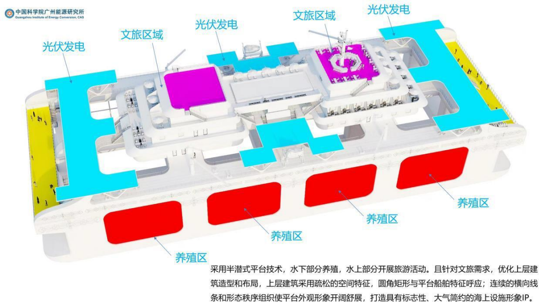
图 3.2.3-6 多功能养殖网箱结构图
