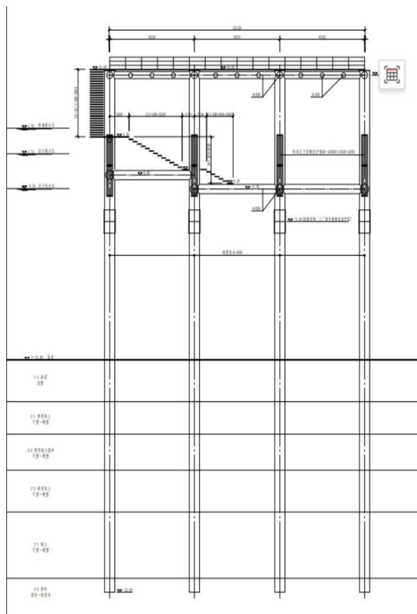
图 3.3.3-5 大型生态养殖围栏平台立面图 (比例 1:100)
