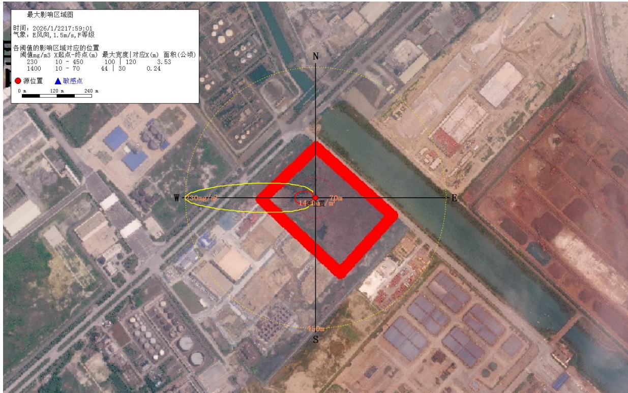
图 6.4-13 异丁醛泄漏最大影响范围图（最不利气象条件）
