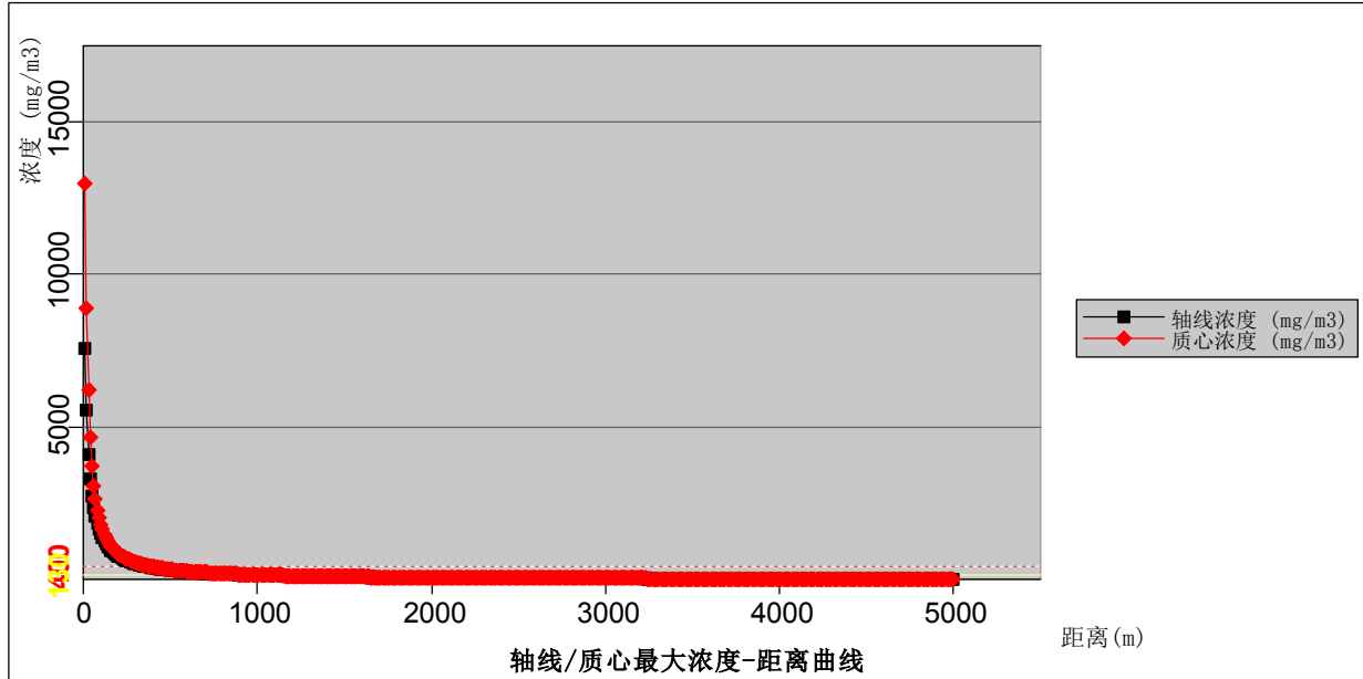
图 6.4-6 氢溴酸下风向轴线最大浓度随距离分布情况（最不利气象条件）
