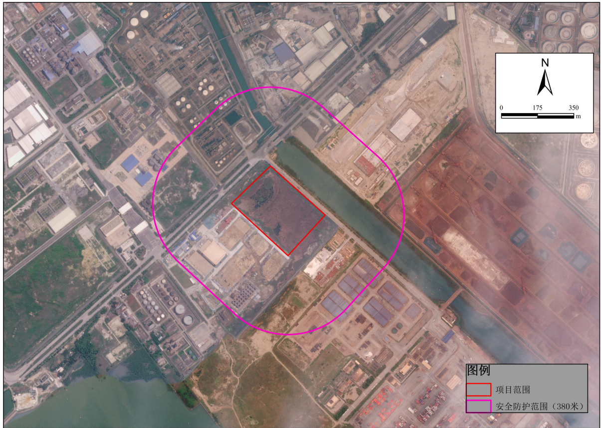
图 6.5-1 项目安全防护范围图
