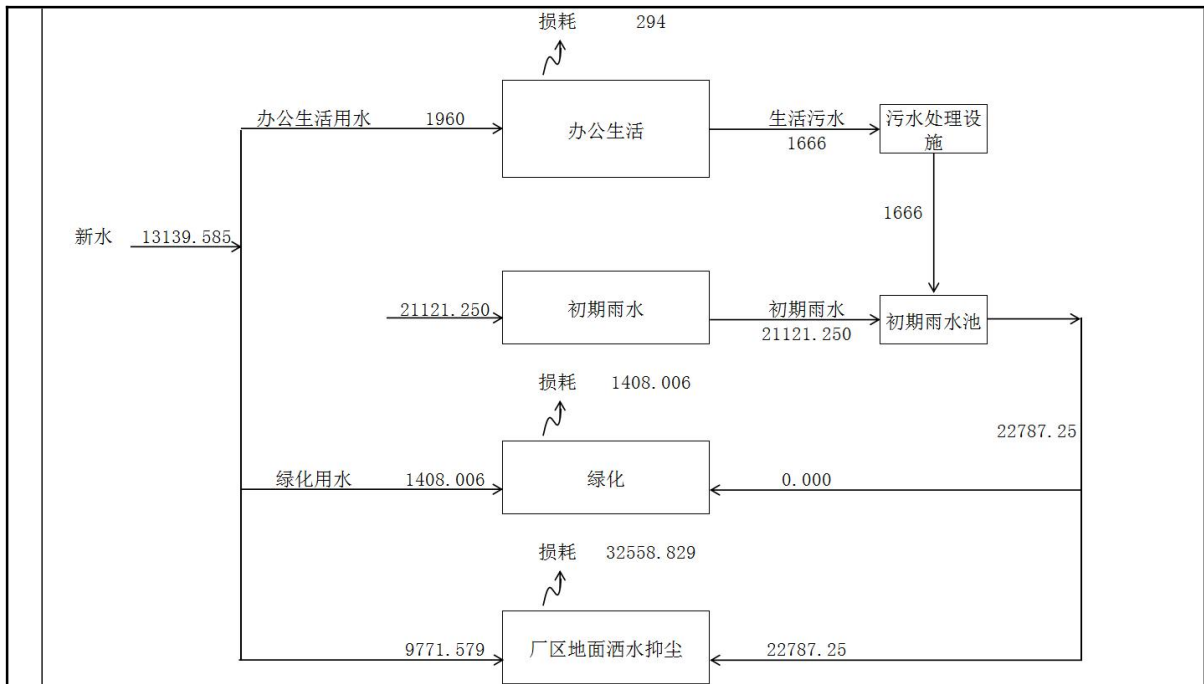
图 4.2.2-3 项目二期建成后全厂水平衡图 (单位: \text{m}^3/\text{a} )
