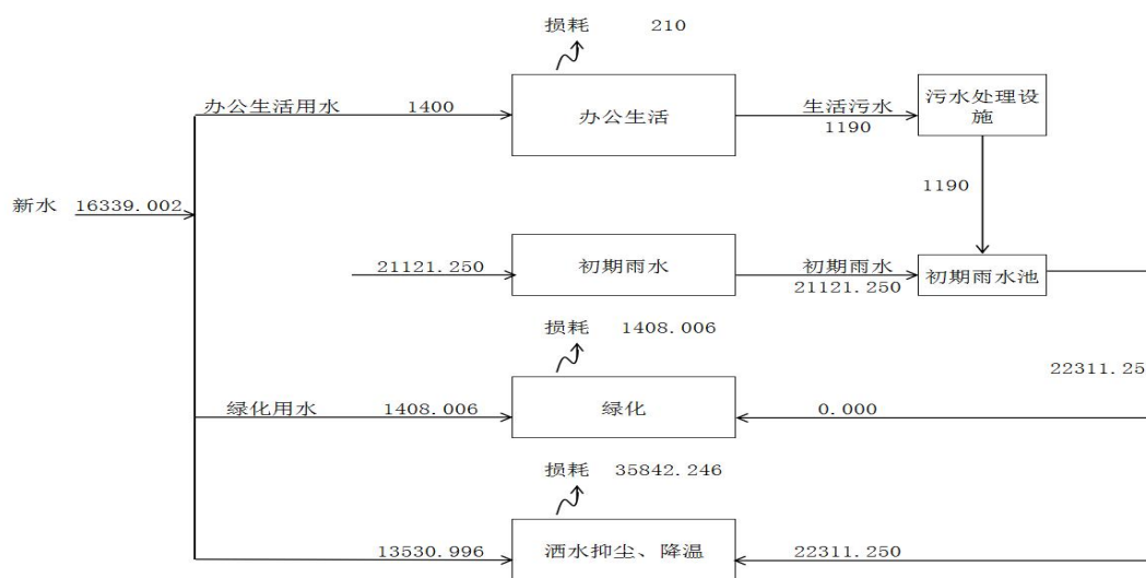
图 4.2.2-2 项目一期水平衡图 (单位: m^3/a )
