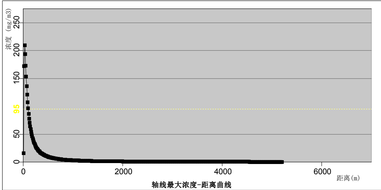
图 6.4-17 CO 下风向轴线最大浓度随距离分布情况（最不利气象条件）
