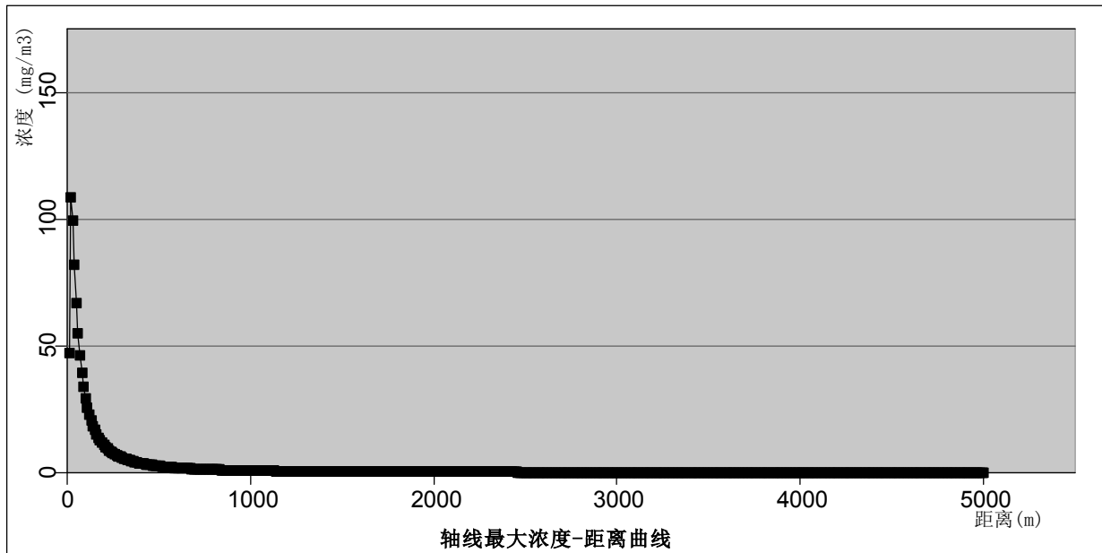
图 6.4-9 丙烯酸正丁酯下风向轴线最大浓度随距离分布情况（最不利气象条件）
