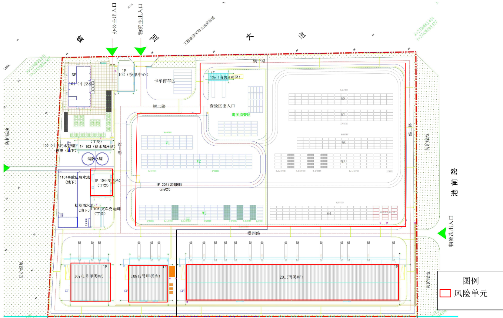
图4.2-1 本项目环境风险单元分布图
