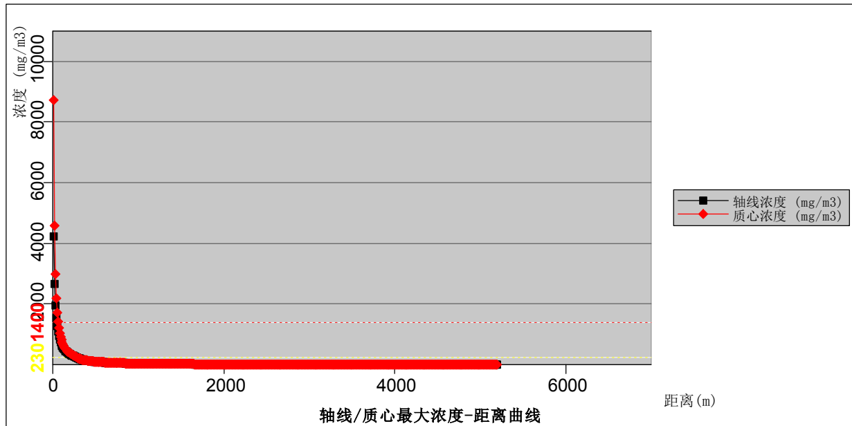
图 6.4-12 异丁醛下风向轴线最大浓度随距离分布情况（最不利气象条件）
