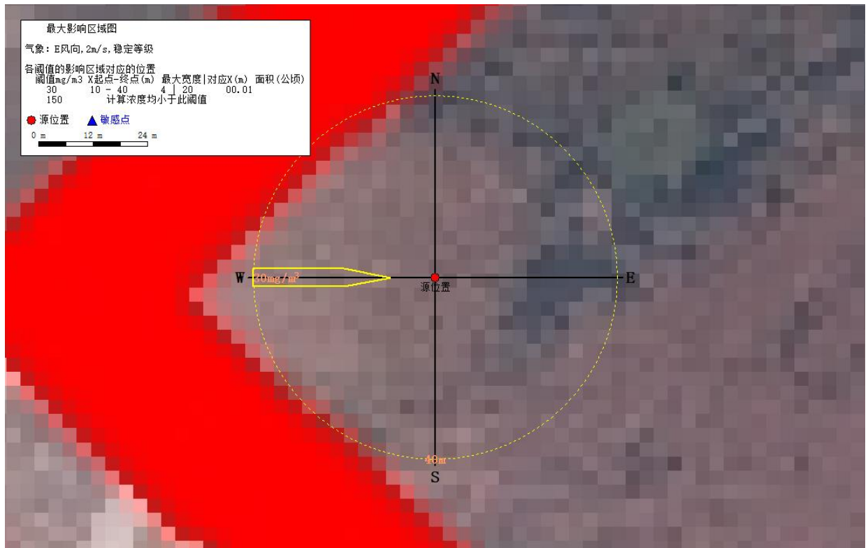
图 6.4-2 正磷酸泄漏最大影响范围图（最不利气象条件）
