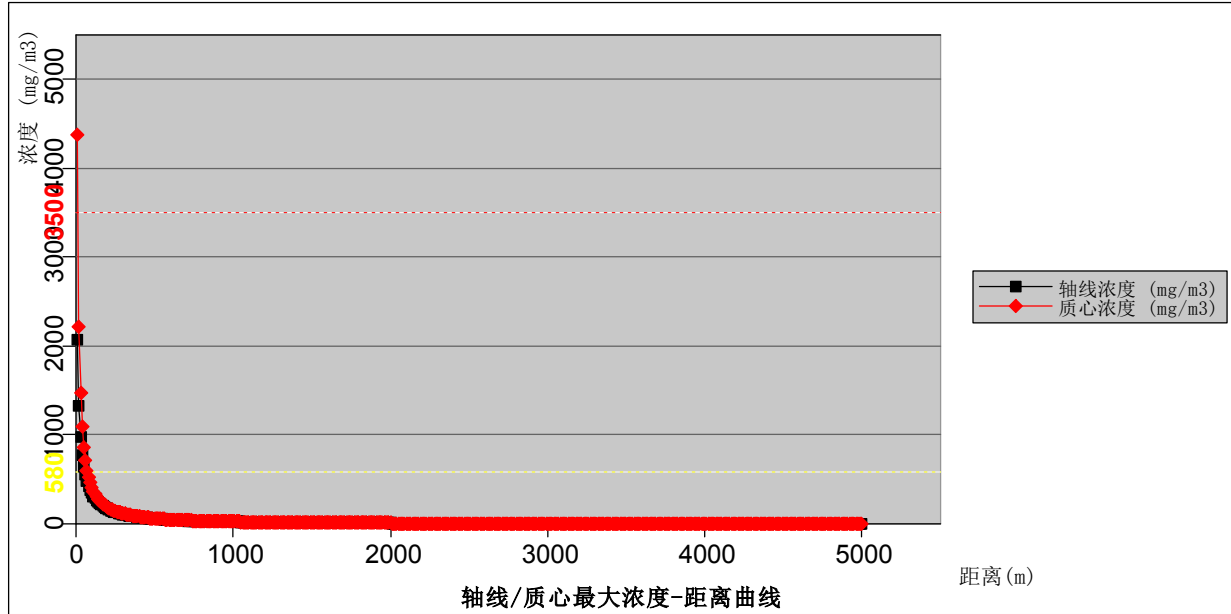
图 6.4-15 丙烯酸甲酯下风向轴线最大浓度随距离分布情况（最不利气象条件）
