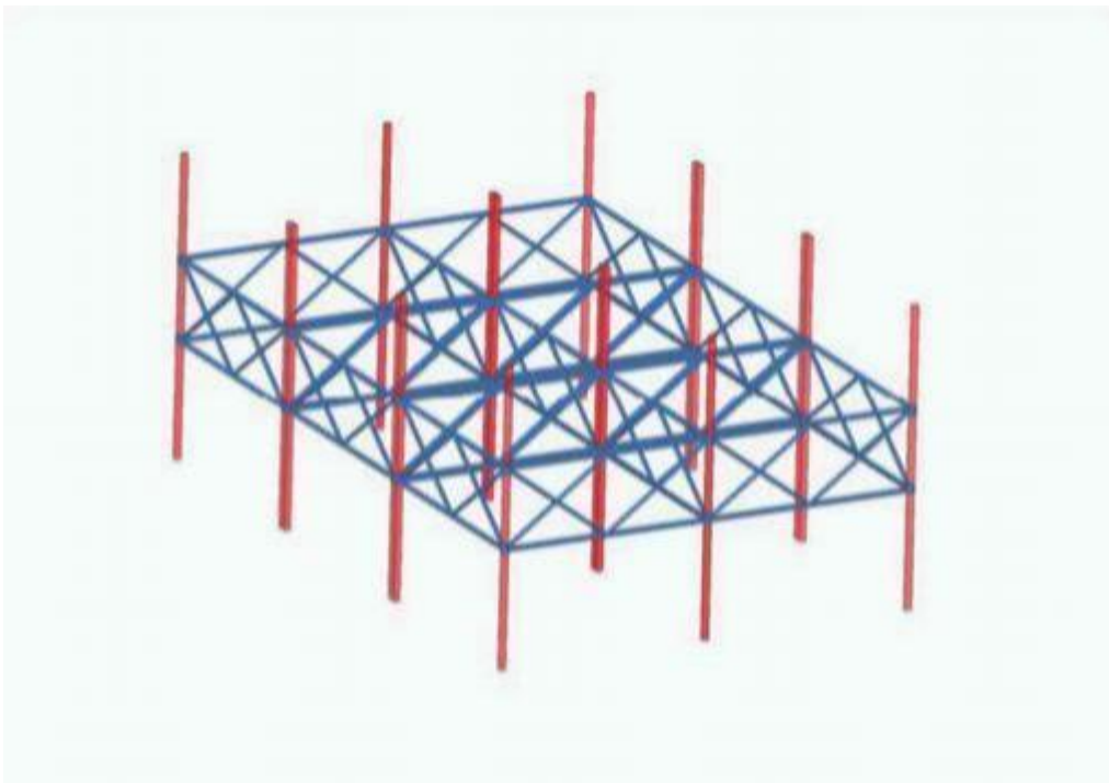
图 3.5-2 整体示意图
