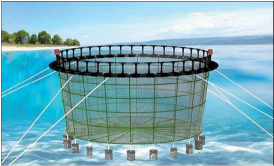
图 3.4-2 单口HDPE 浮式圆形重力式深水网箱立体结构示意图
