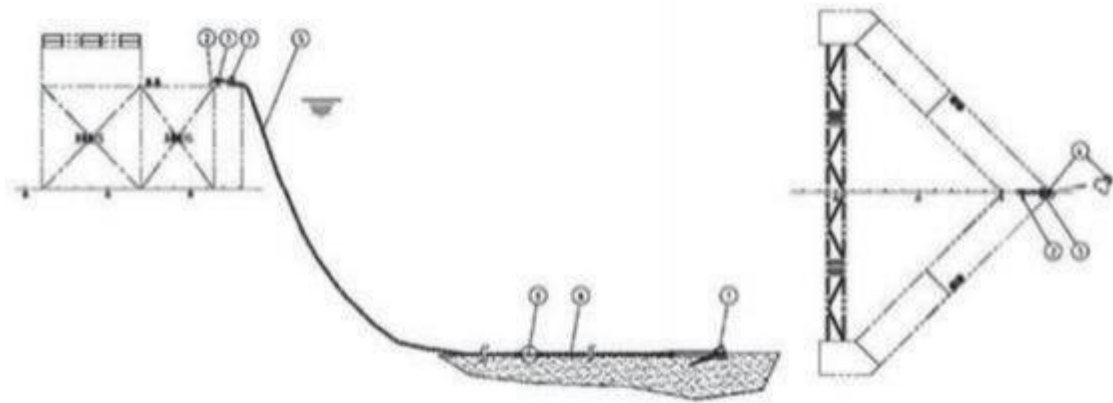
图 3.4-8 锚链结构图
