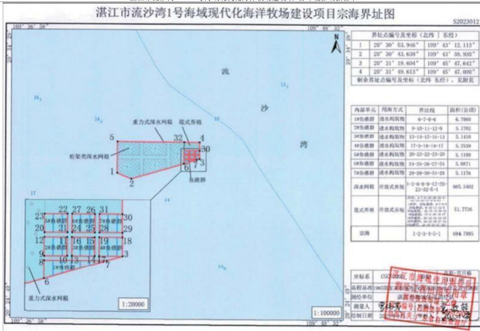
图 3.9-2 宗海界址图
