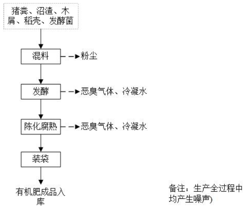
图 3.3-4 有机肥生产工艺流程示意图
