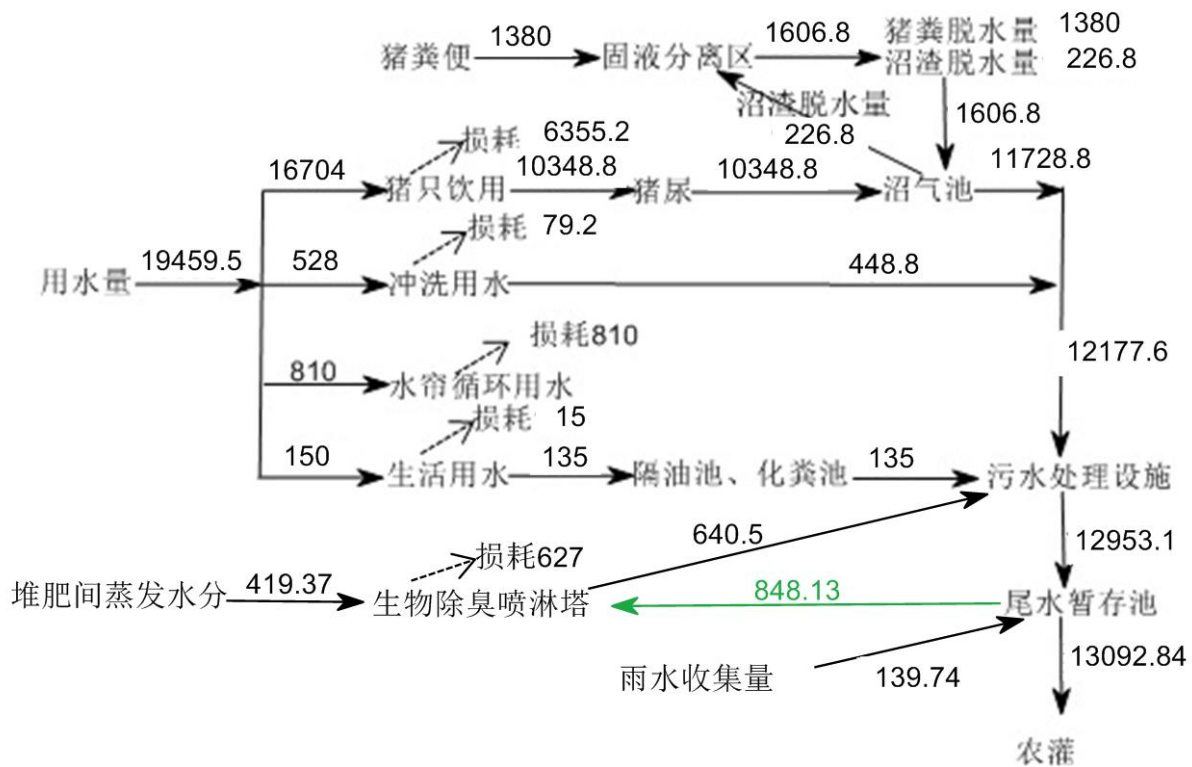
图 3.3-6 项目水平衡图
