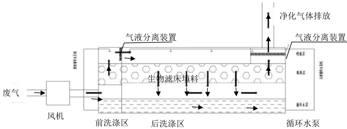
图 3.3-5 生物除臭喷淋塔工艺图
