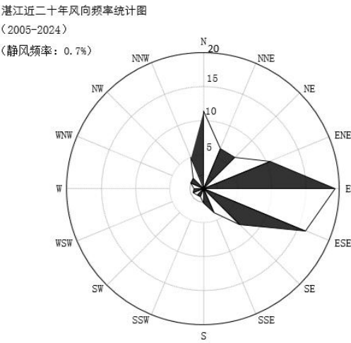
图 5.2.1-3 湛江市近 20 年风向玫瑰图
