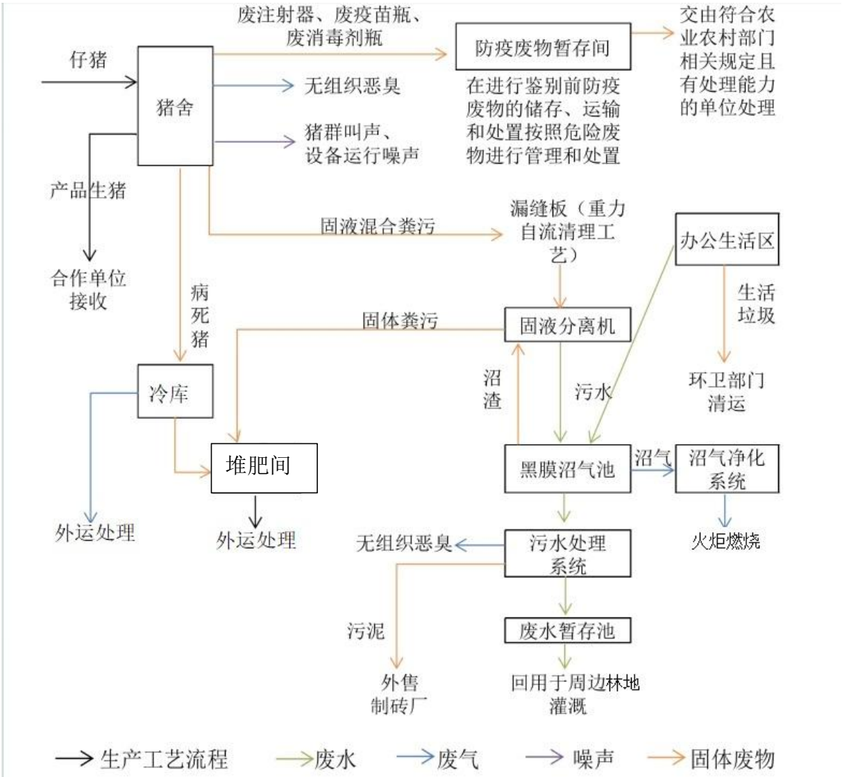
图 3.3-1 项目生产工艺总流程图
