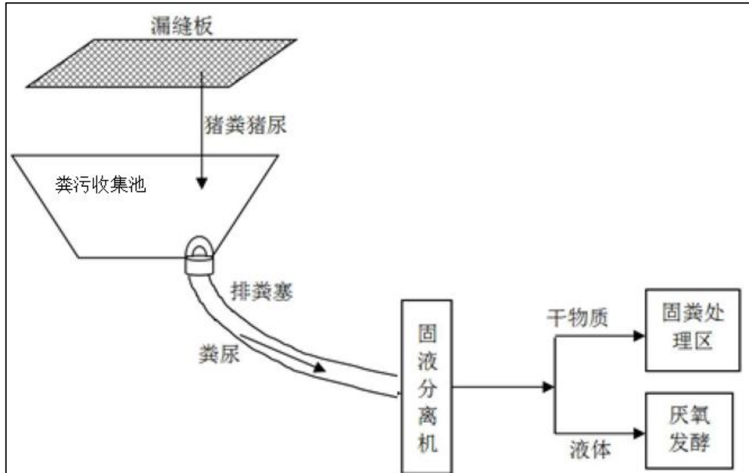
图 3.3-2 本项目清粪工艺示意图
