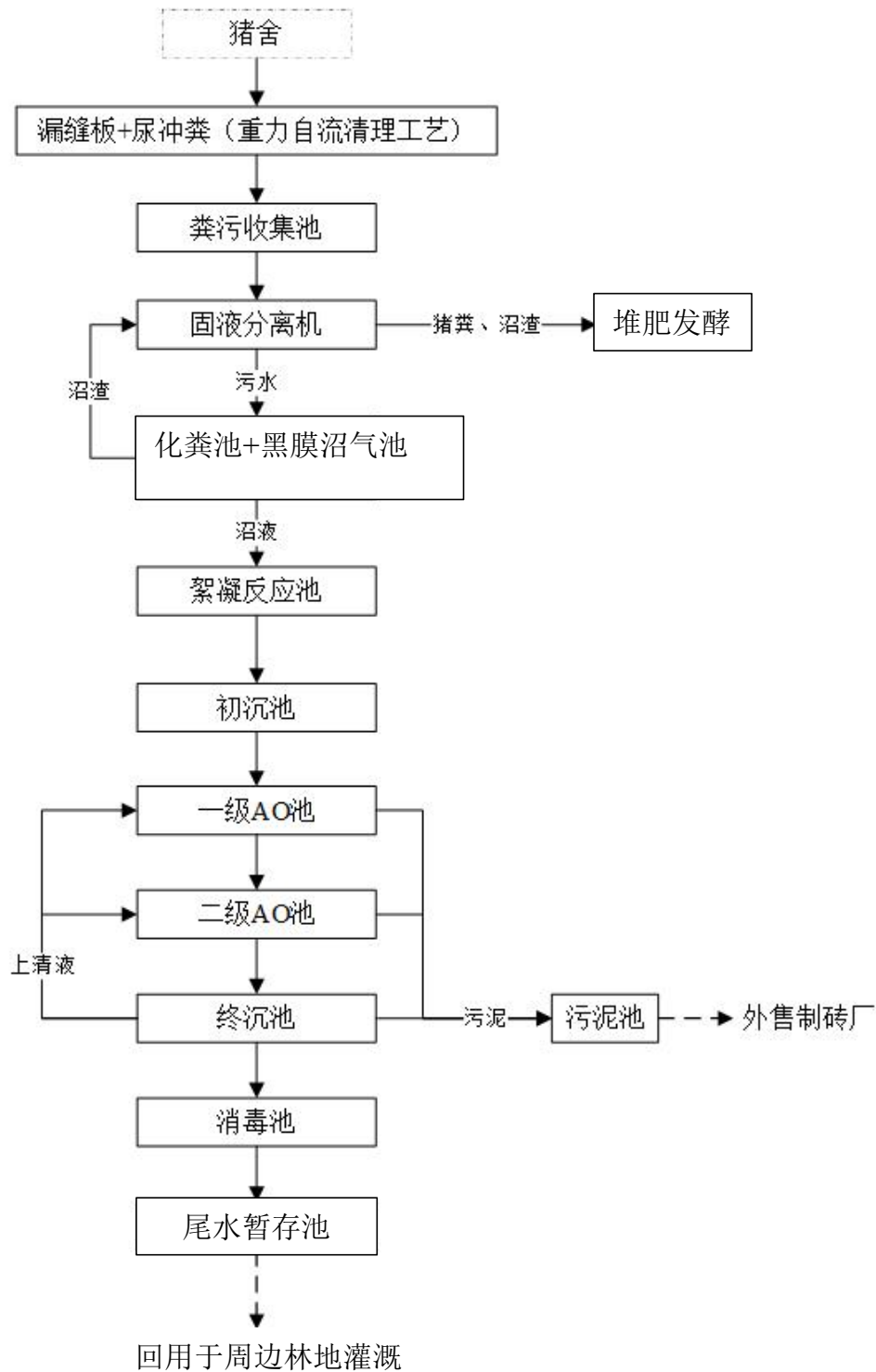
图 3.3-3 废水处理工艺流程示意图
