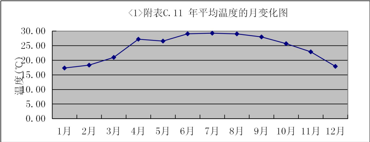
图 5.2.1-4 湛江市 2024 年各月平均温度变化曲线图
