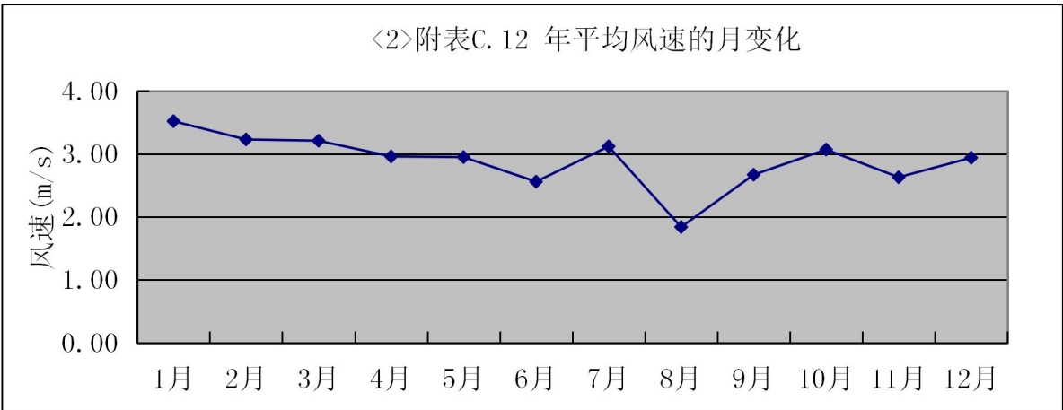
图 5.2.1-5 湛江市 2024 年各月平均风速变化曲线图
