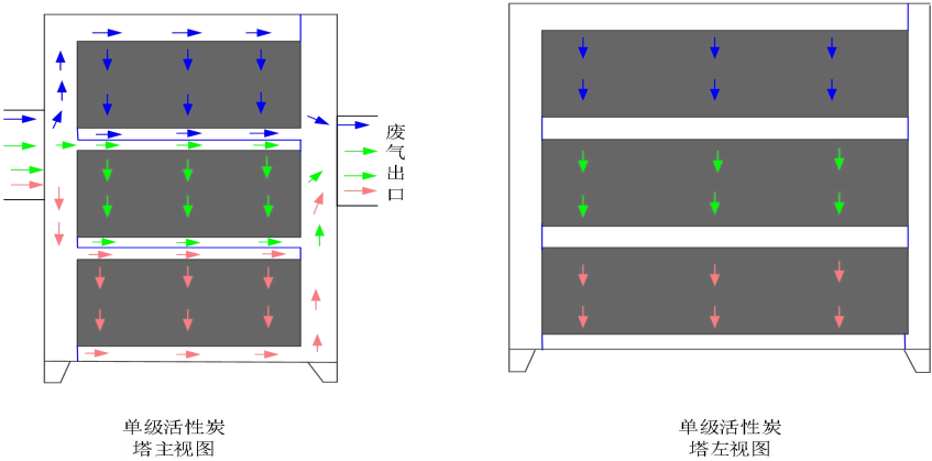
图 4-1 单级活性炭箱内部结构示意图（3 层）
