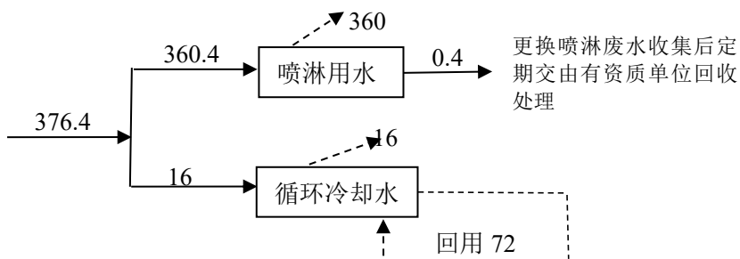
图 2-2 项目近期水平衡图 单位： \text{m}^3/\text{a}
