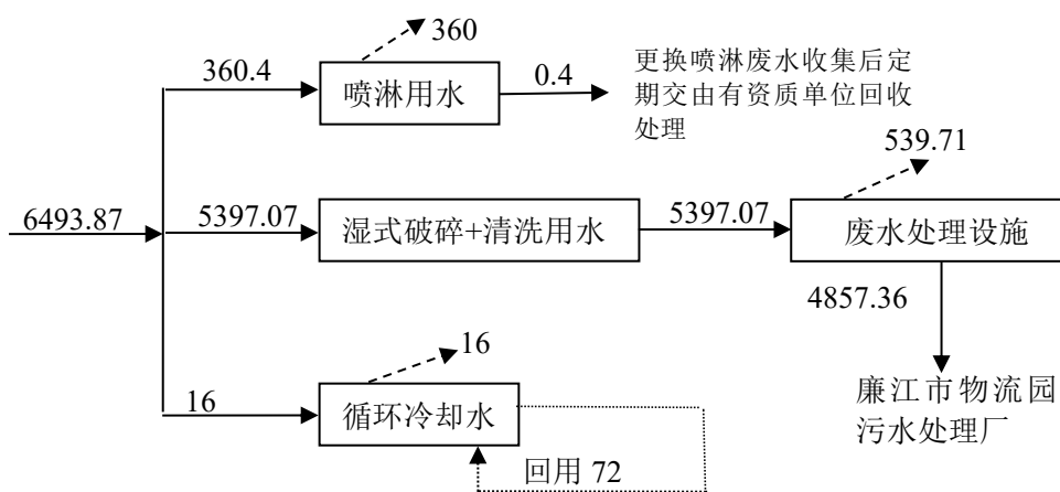
图 2-2 项目远期水平衡图 单位： \text{m}^3/\text{a}
