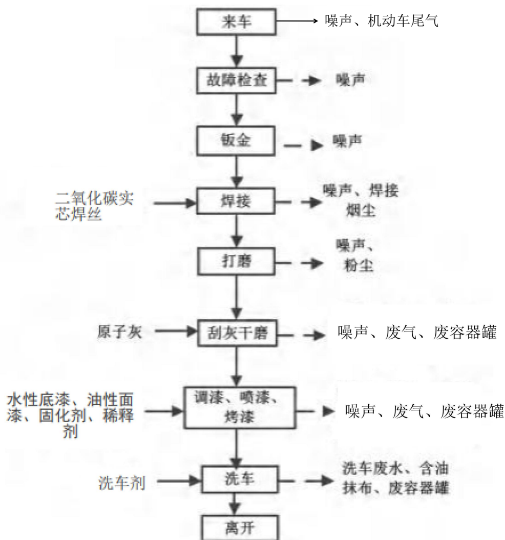
图 2-6 汽车修理与维护工艺流程图
