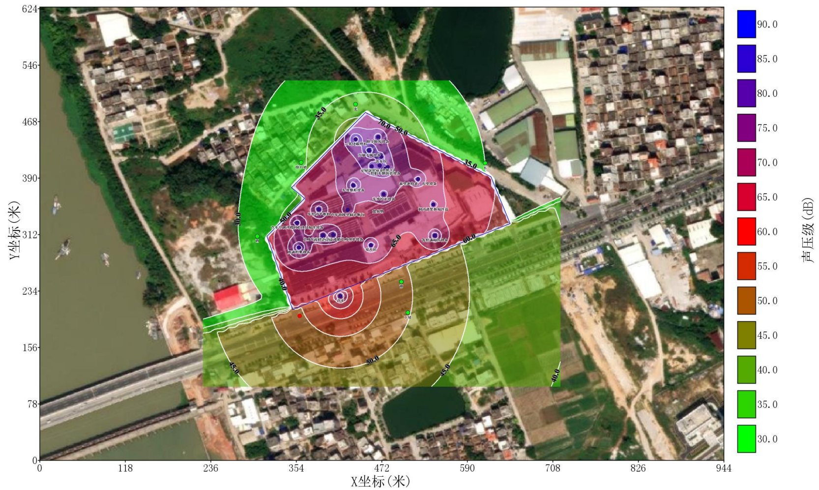
图 4-1 项目等声级线图
