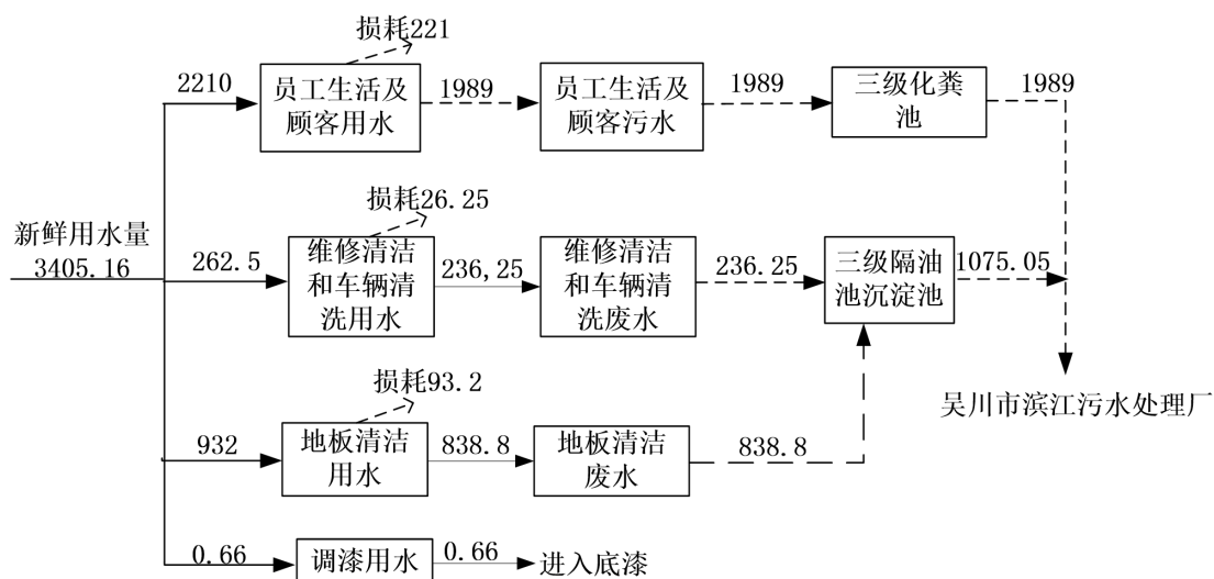
图2-1 改扩建后全厂水平衡图（单位：m 3 /a）
