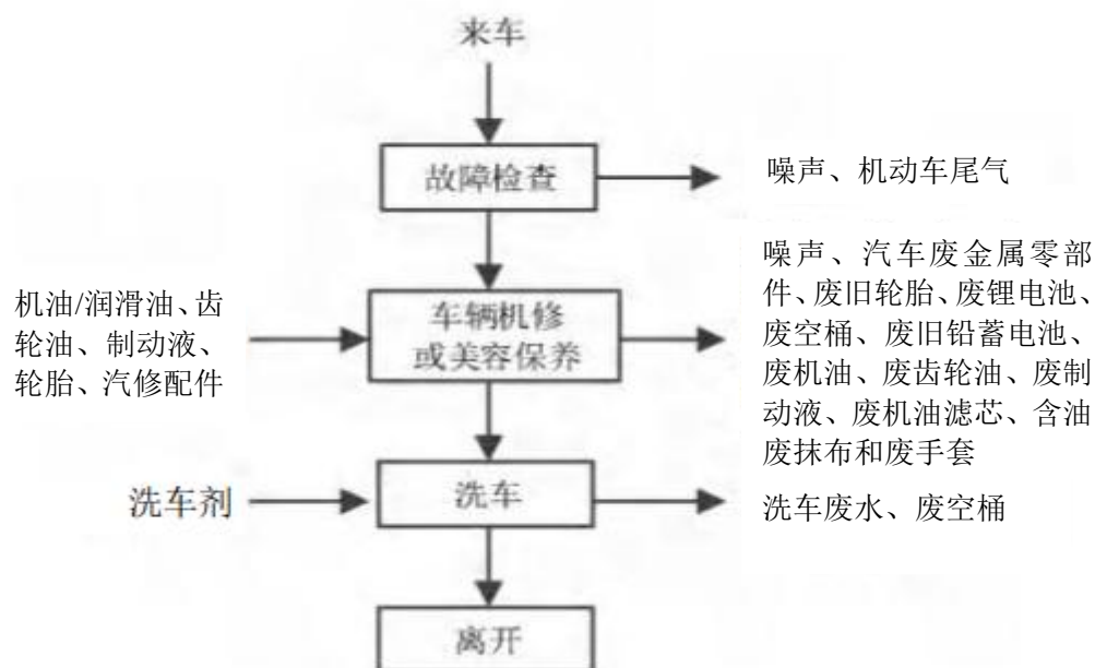
图 2-5 汽车机修、美容保养工艺流程图
