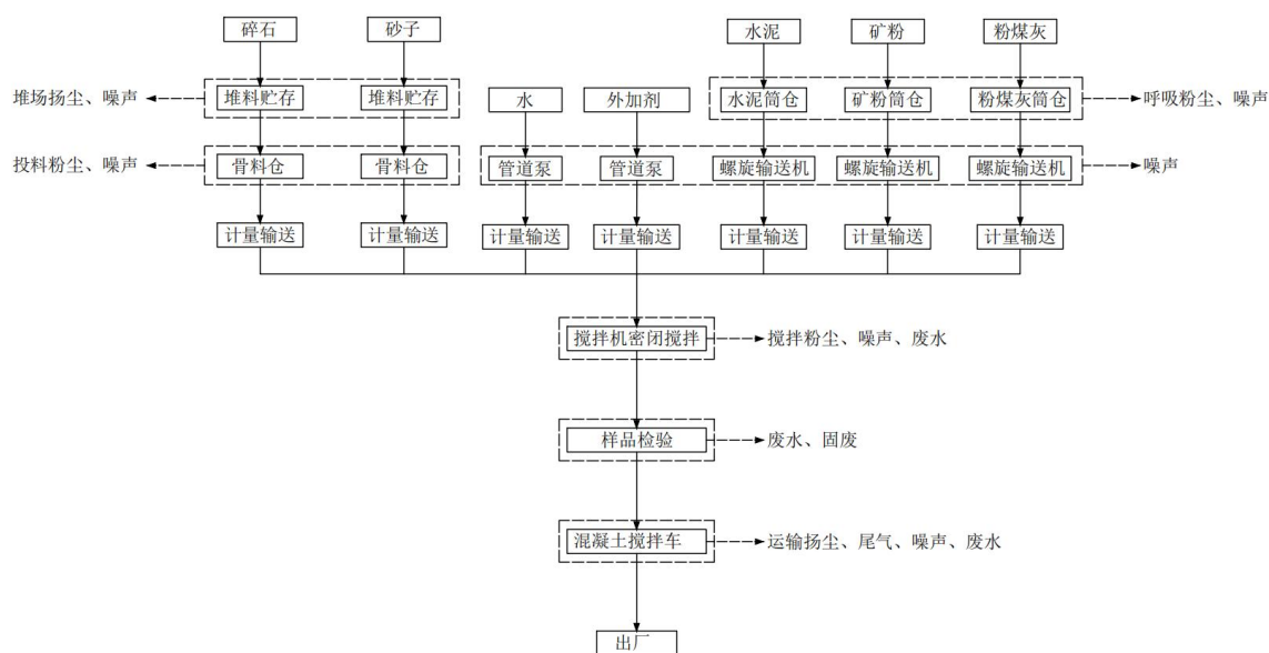
图 2-2 生产工艺流程及产污示意图
