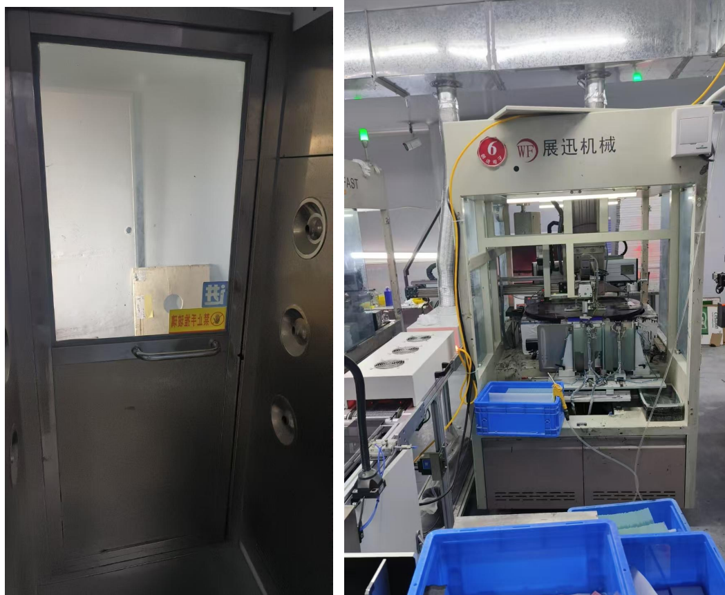
图 4-2 密闭缓冲区示意图&丝印机收集示意图
