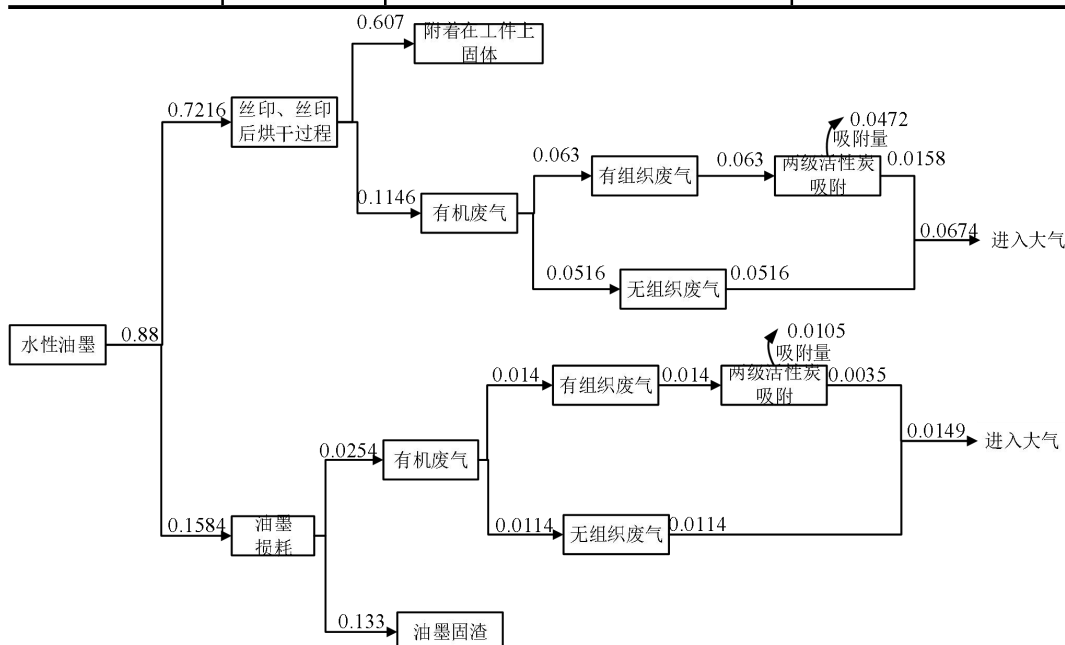
图2-1 水性油墨平衡图 单位:t/a
