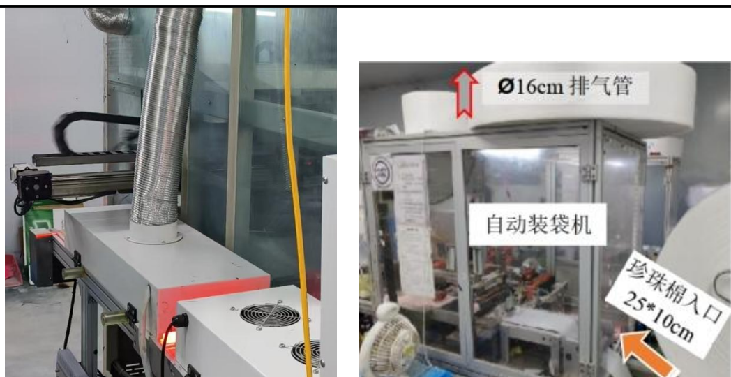
图 4-3 烘干机&包装机收集示意图
