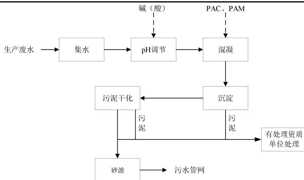
图4-6 厂区内污水处理设施工艺流程
