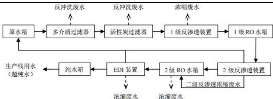
图2-5 纯水制备工艺流程图
