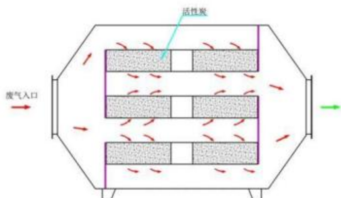
图 4-4 单级活性炭箱内部结构示意图(3 层)
