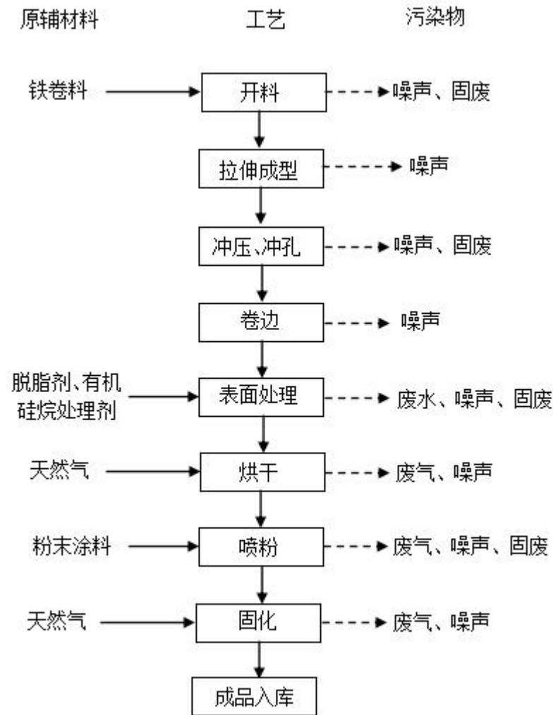
图 2-2 生产工艺流程及产排污环节示意图
