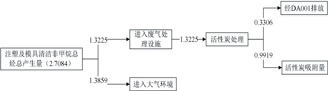
图 3 改扩建后项目 VOCs 平衡图（t/a）
