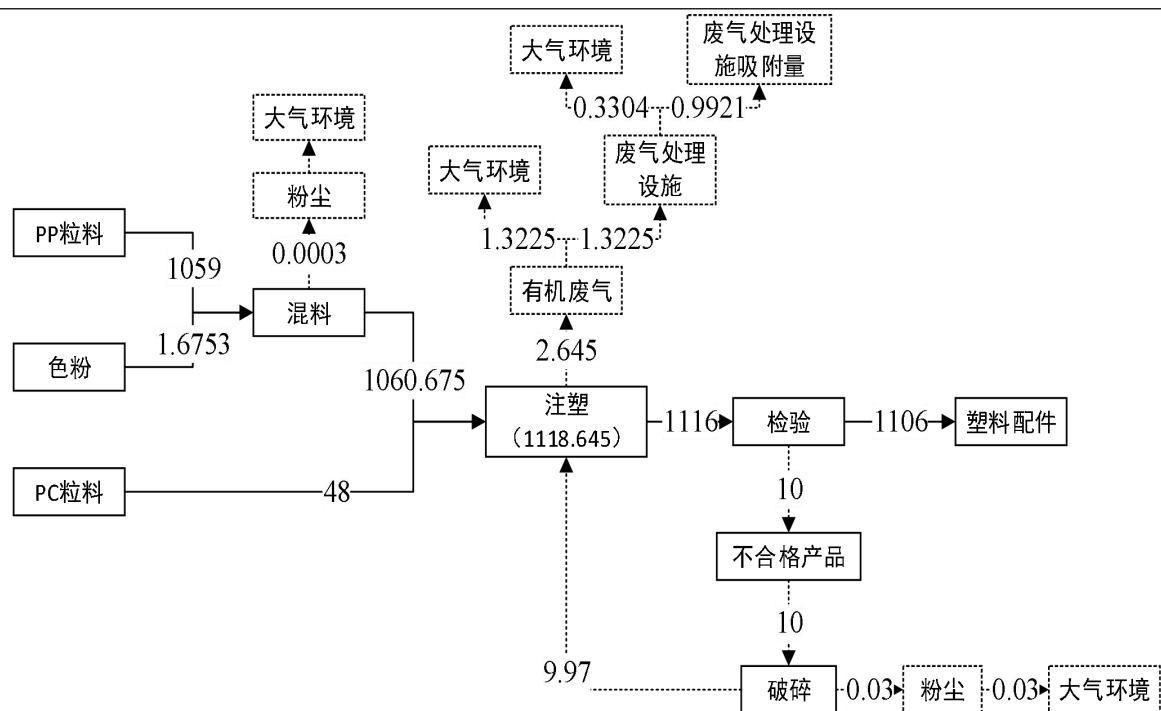
图4 改扩建后项目注塑工序物料平衡图（t/a）
