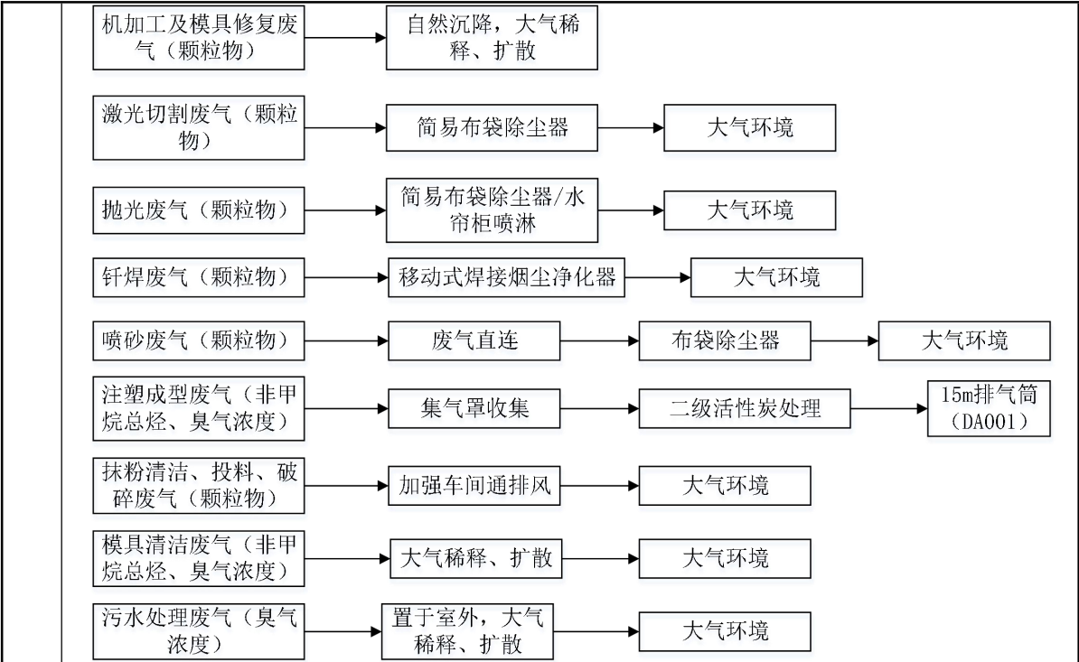
图 11 项目废气处理工艺流程图
