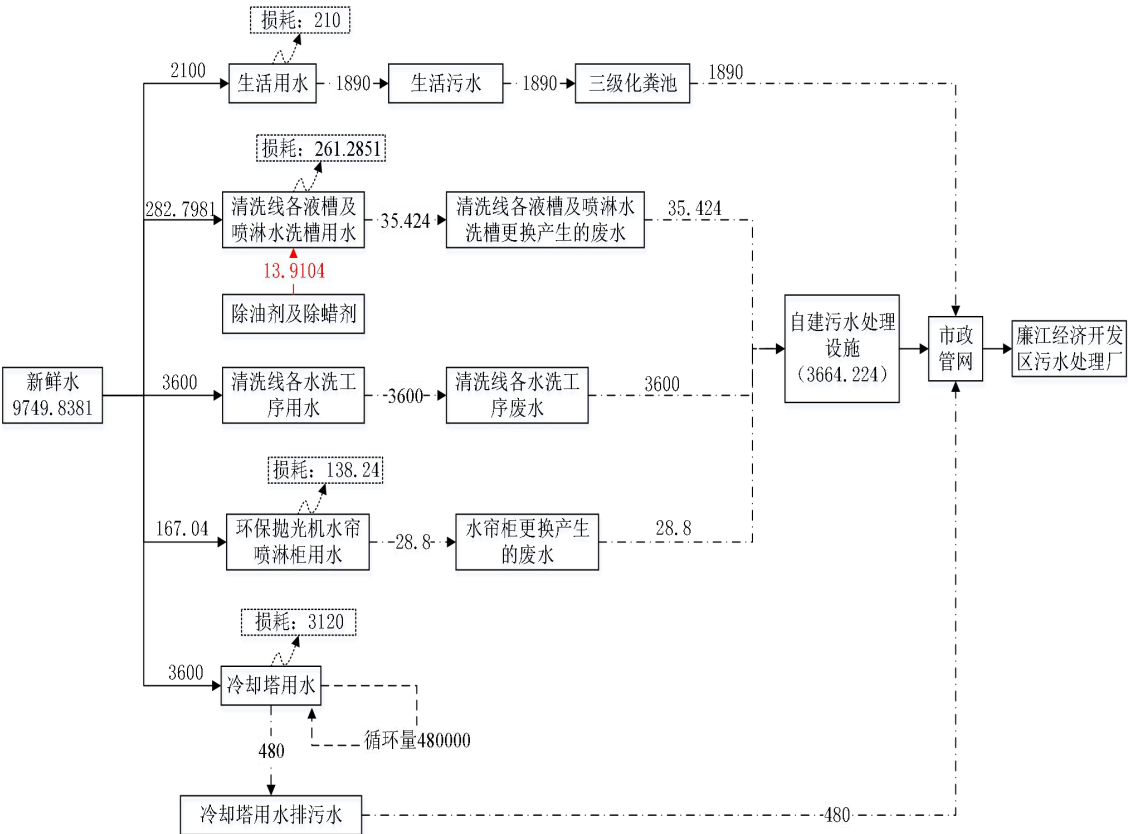
图 2 改扩建后项目水平衡图 (t/a)
