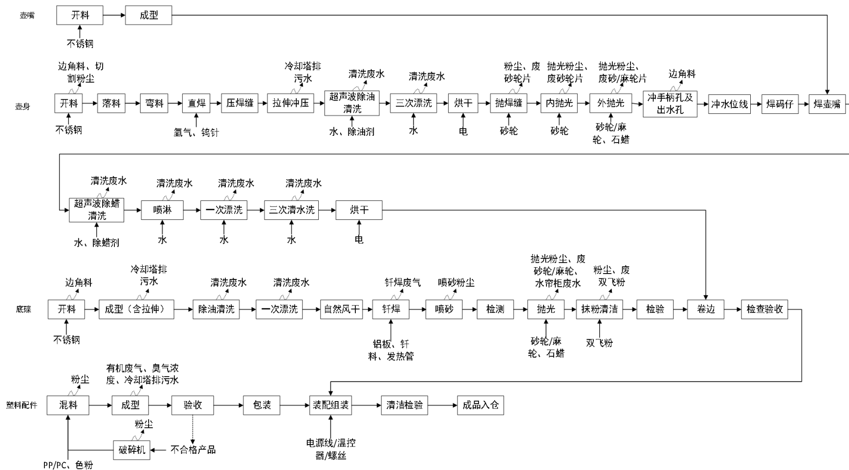
图 5 改扩建后项目生产工艺流程图
