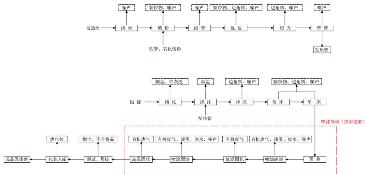
图 2-4 营运期发热盘工艺流程及产污示意图
