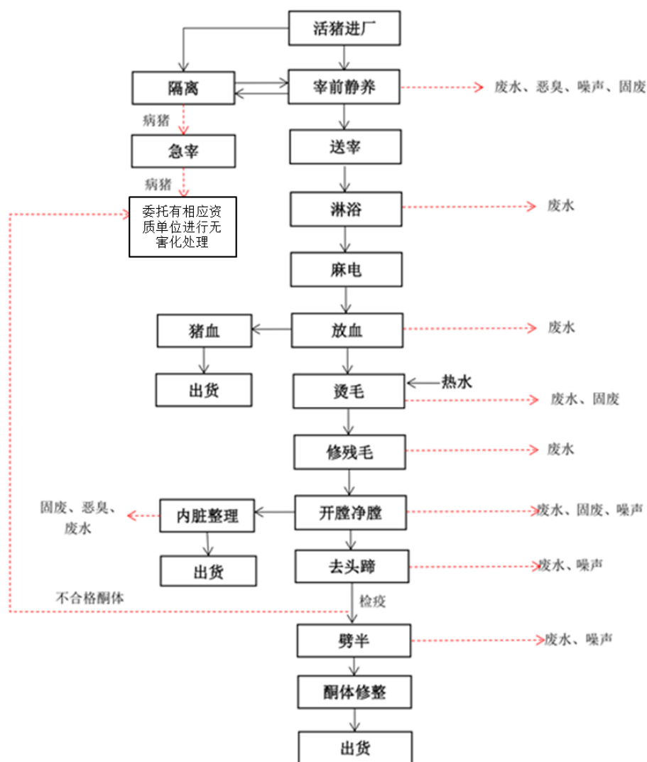
图 2-2 本项目生猪屠宰工艺流程图
