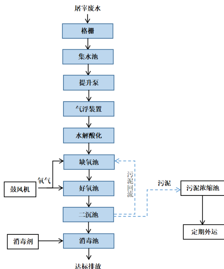
图 4-1 污水处理工艺流程
