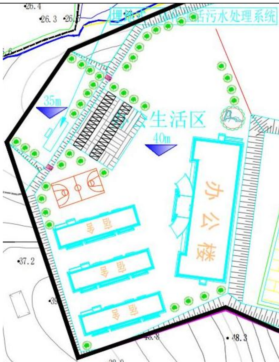
图 2-8 办公生活区平面布置图
