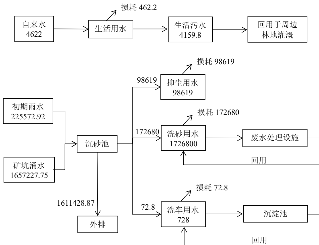
图 2-3 水平衡图 (单位: m³/a)
