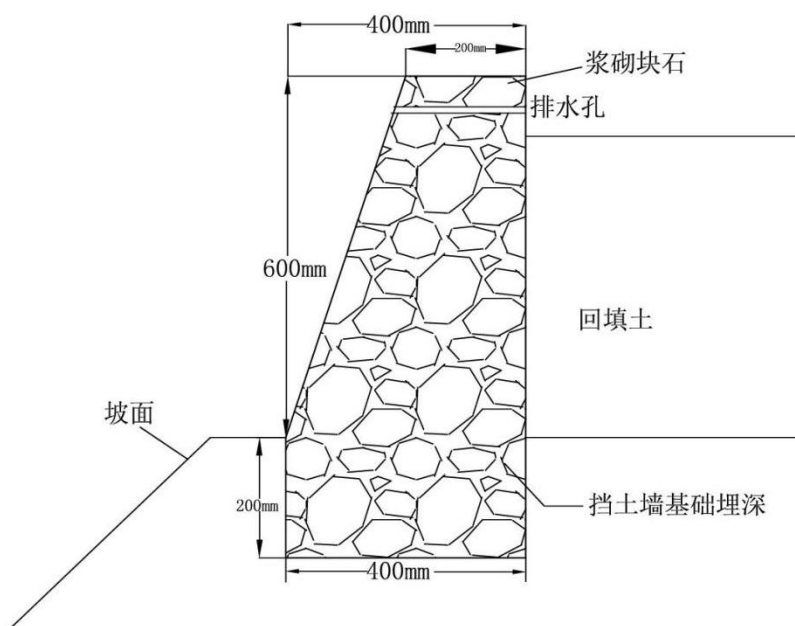
图 5-2 挡土墙结构断面图
