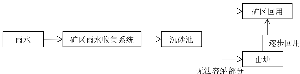
图 4-2 雨水处理工艺流程图
