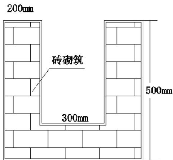
图 5-1 排水沟结构断面图
