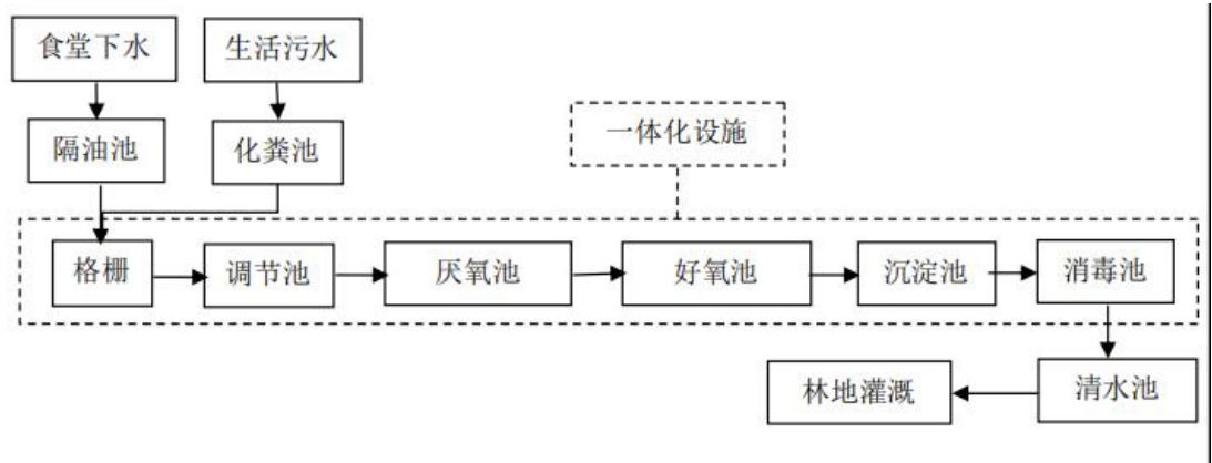
图 5-1 地埋式一体化生活污水处理工艺流程图
