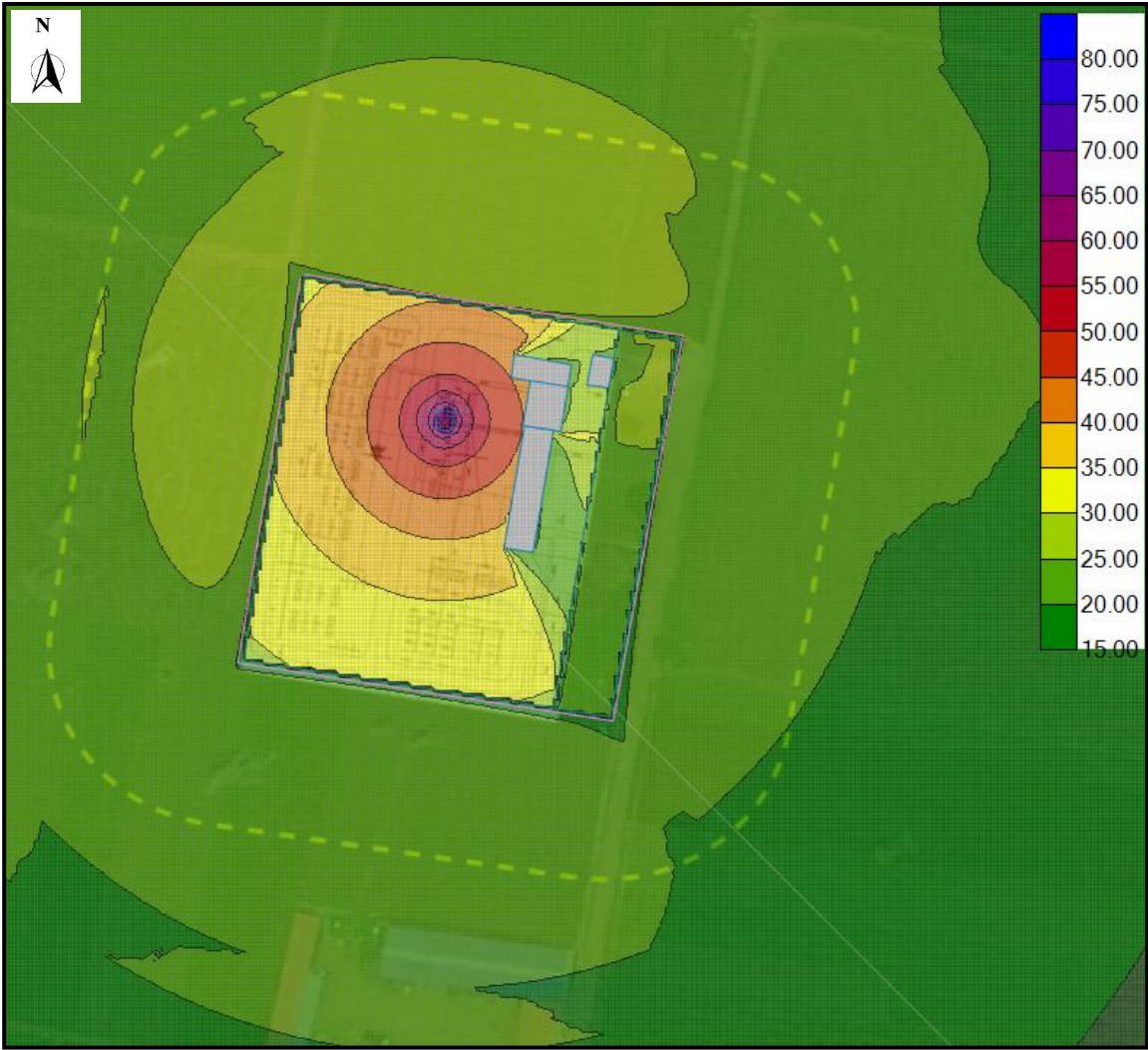
图 4.4-1 噪声贡献值等声级线图
