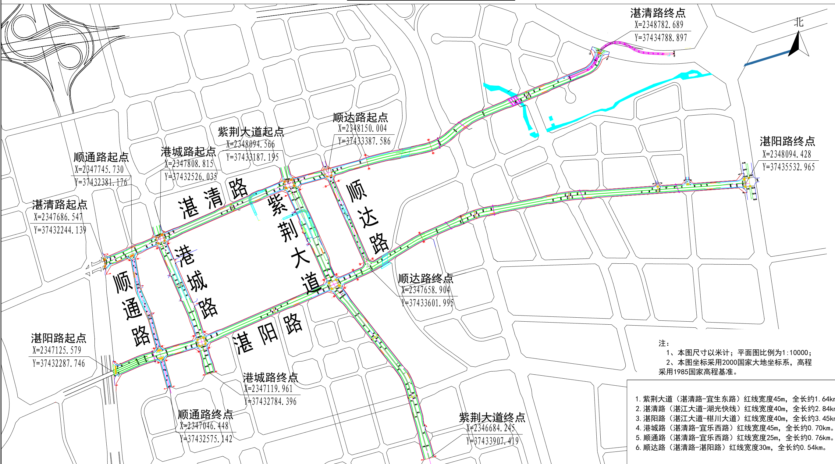
道路平面设计图
