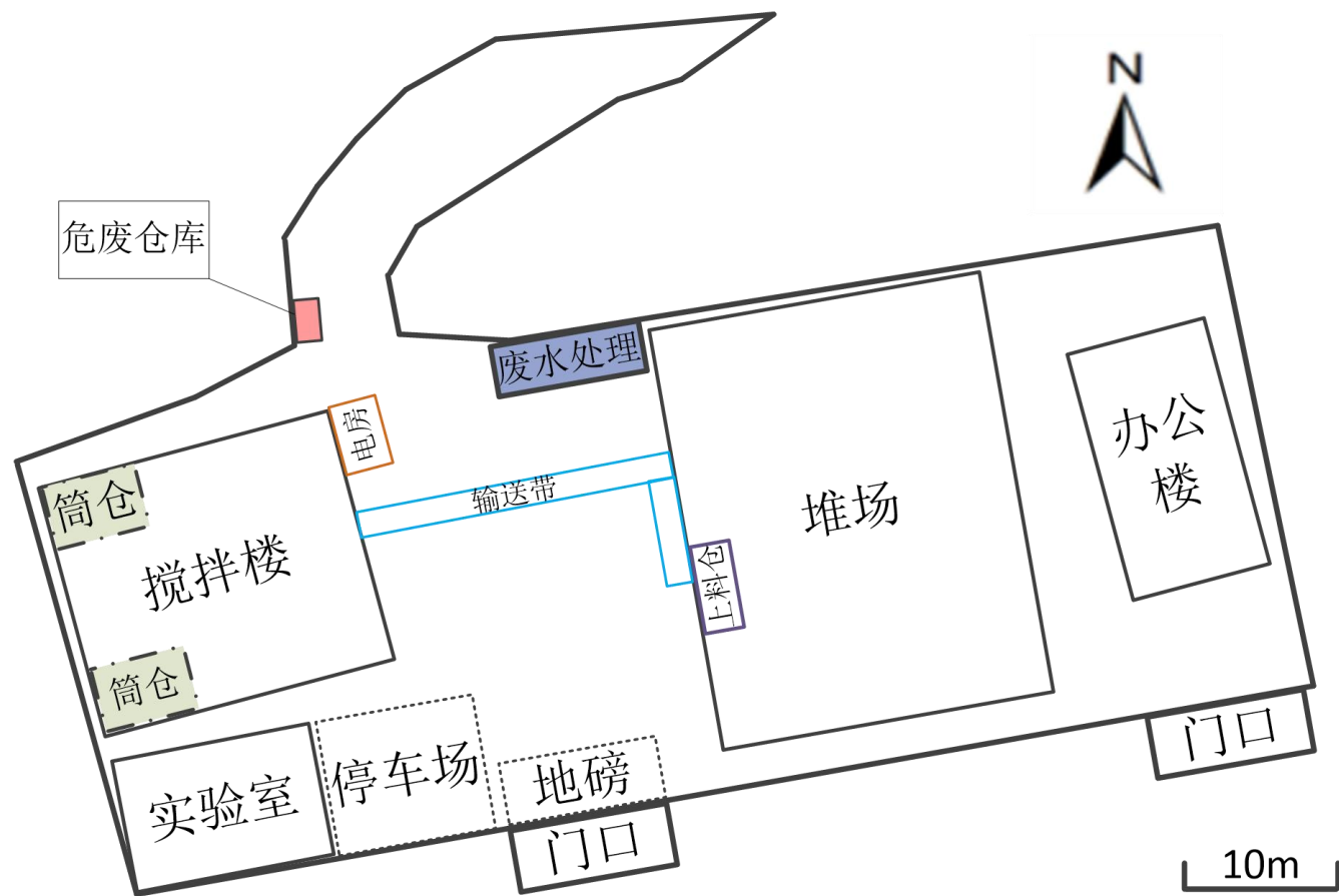
附图4厂区平面布置图
