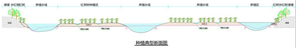
图 3.2.2-17 潮沟开挖及回填典型断面示意图
