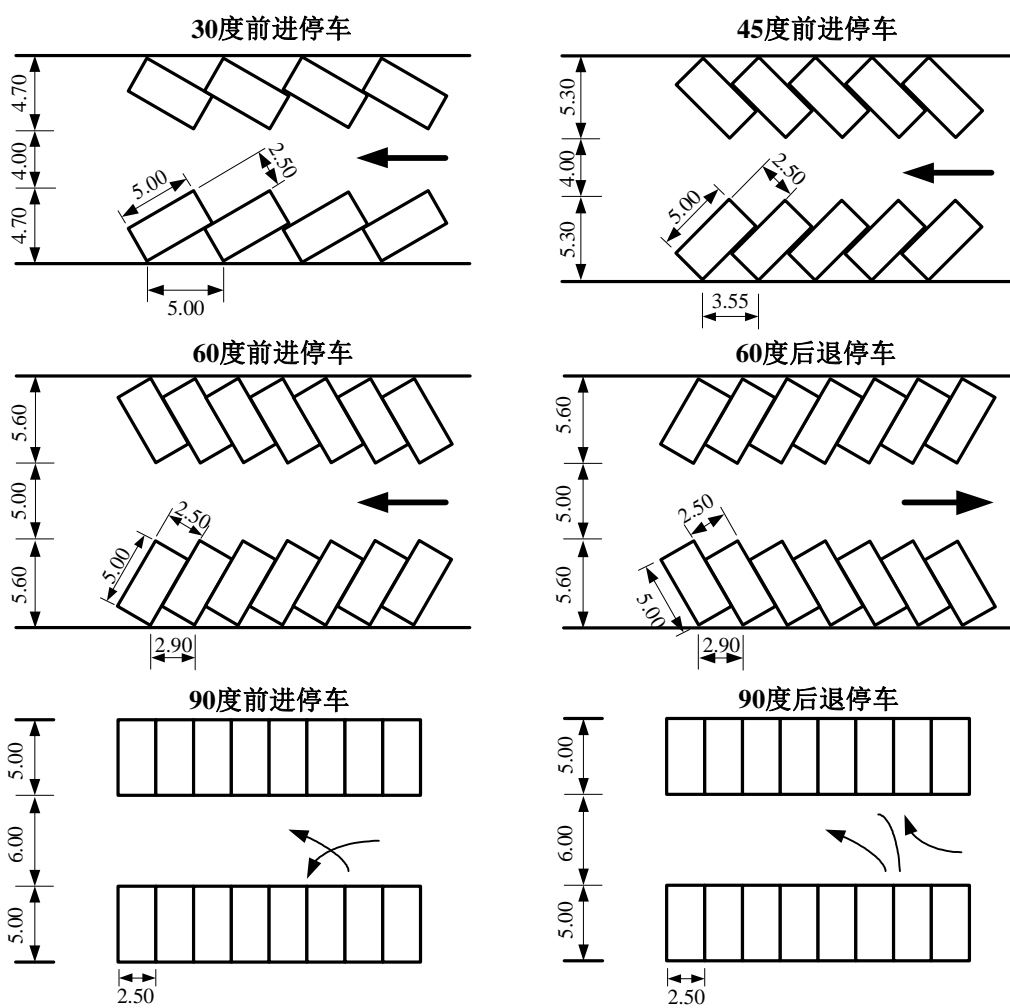
小型车停车方法、停车车位布置图 附图一
